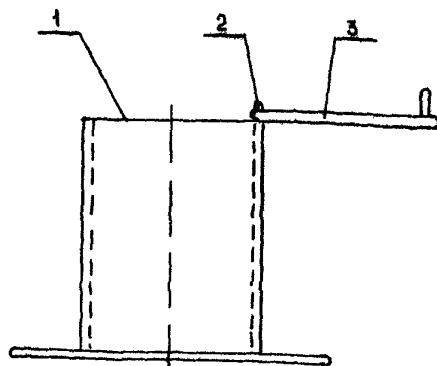
Рис. 7.1 Прибор для определения насыпной плотности сыпучего груза 1 - мерный сосуд; 2 - штатив; 3 - поворотная рамка
