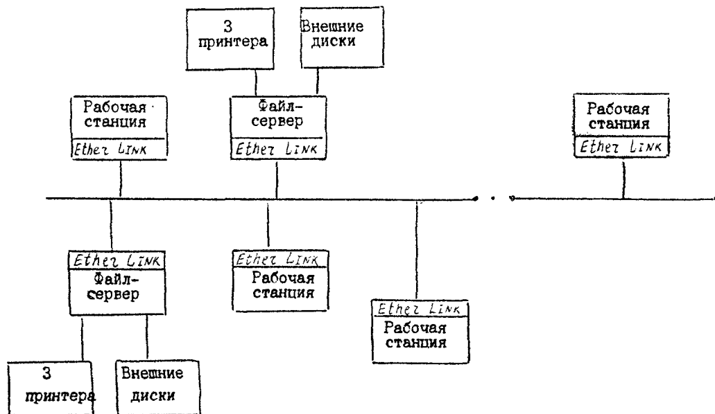
Рис. 4.3 Схема сети типа ETHERNET
