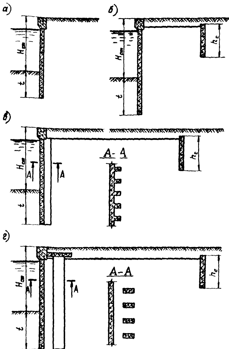
Рис 1 Схемы сооружений а-незаанкеренный болюверк; б, в-заанкеренный болюверк; в-экрани- рованный заанкеренный болюверк
