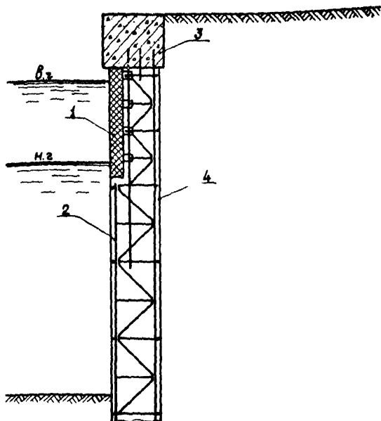
Рис. 4. Вариант балковки с плитой из термопластичного материала:
