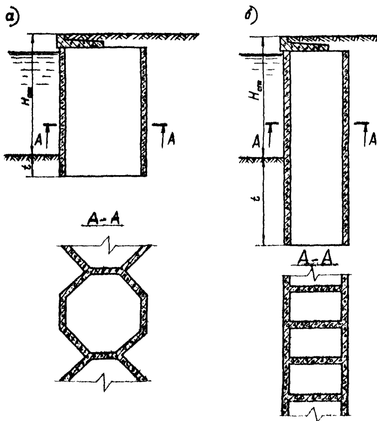
Рис. 2. Сооружения ячеистого типа: а-гравитационное; б-гравитационное затопленное
