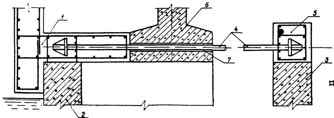
Рис 5 Крепление анкера: табрового сечения ; 1- железобетонная накладка; 2- лицевая стенка 3- анкерная стенка; 4- анкер; 5- оголовок анкерной стенки; 6- паркановая балка; 7- труба
