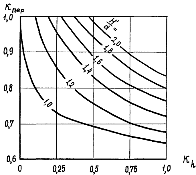
Рис. 4.I2. График для определения коэффициента k_{пер}
