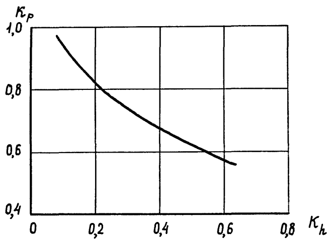
Рис.4.II. График для определения коэффициента k_p .
