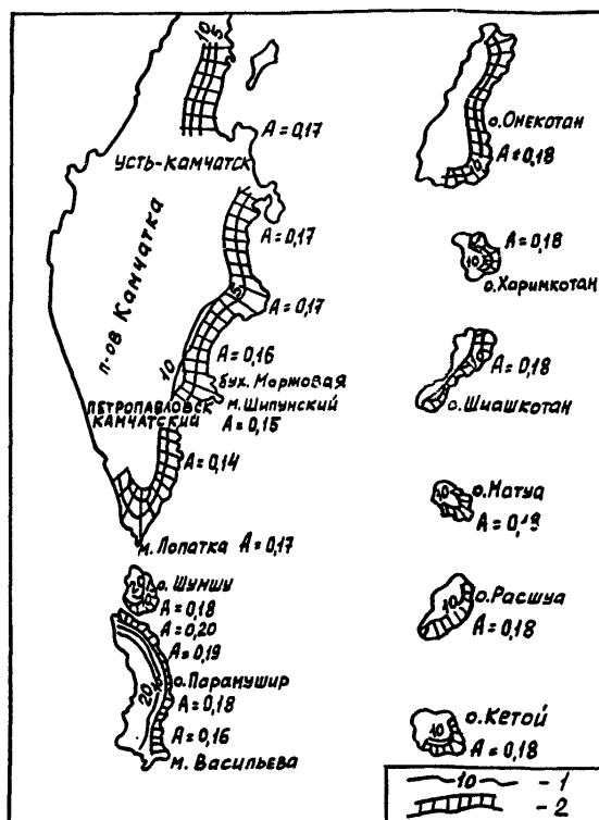
Рис. 2.1 Схема районирования Тихоокеанского побережья Камчатки и Курильских островов по параметру A (г-I) и h_{100} (м). Условные обозначения: I - условные изогипсы; 2 - h_{100} - уровень максимального подъема воды с 1%-ой обеспеченностью (1 раз в 100 лет)
