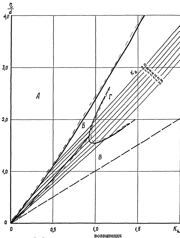
Рис.4.6. График для определения \eta воды перед сооружением \eta . (Пунктиром показана расчетная граница)
