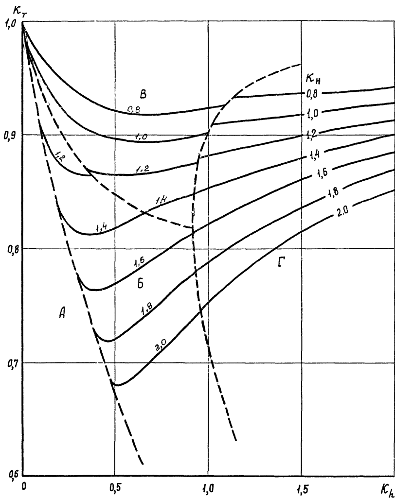
Рис. 4.8. Графики для определения коэффициента ослабления волны пучами, при её взаимодействии с вертикальным сооружением.
