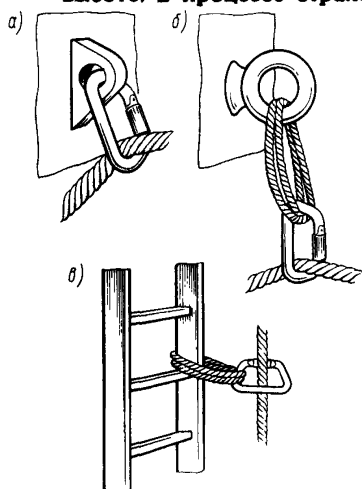
Рис. 3. Организация промежуточных точек страховки: а — непосредственное крепление карабина; б, в — крепление карабина с помощью кренгельс-стропы
