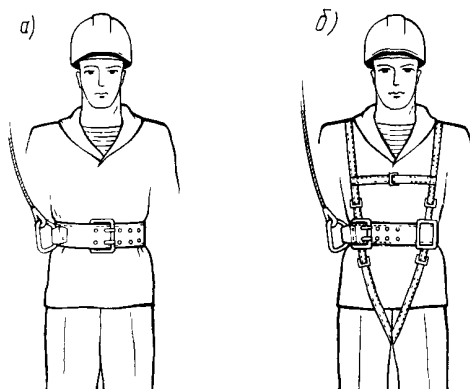
Рис. 2. Конструкции предохранительных поясов:
