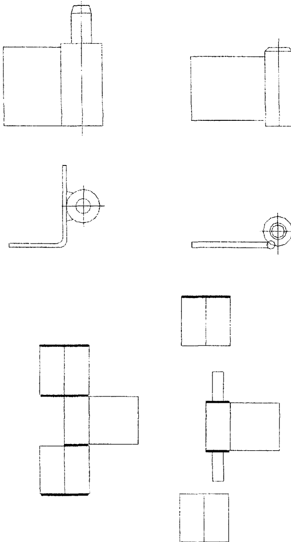
Рисунок Б.2 — Примеры дверных петель
