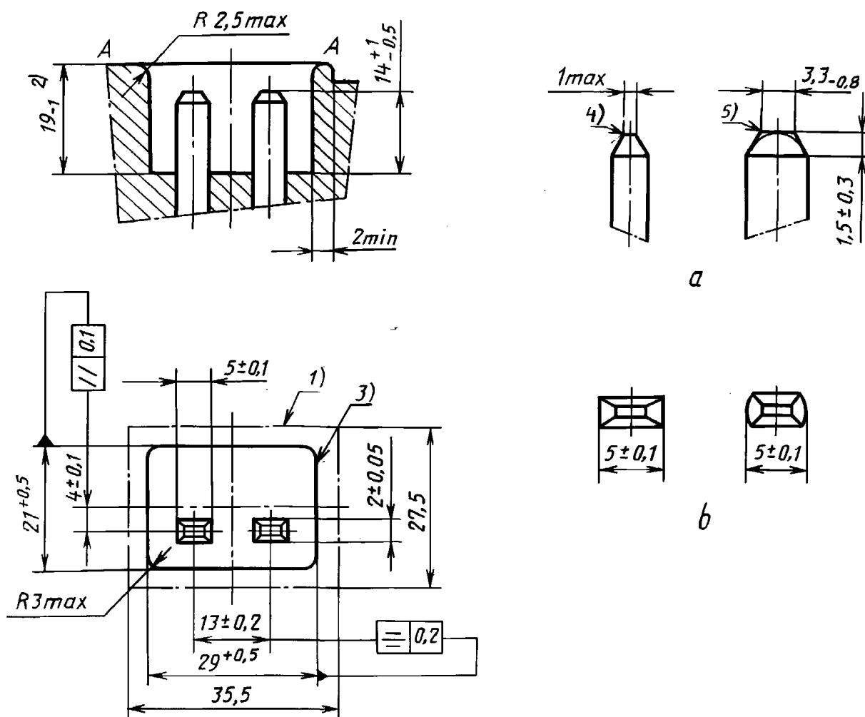
а — вариант исполнения концов штырей; б — варианты формы штырей
