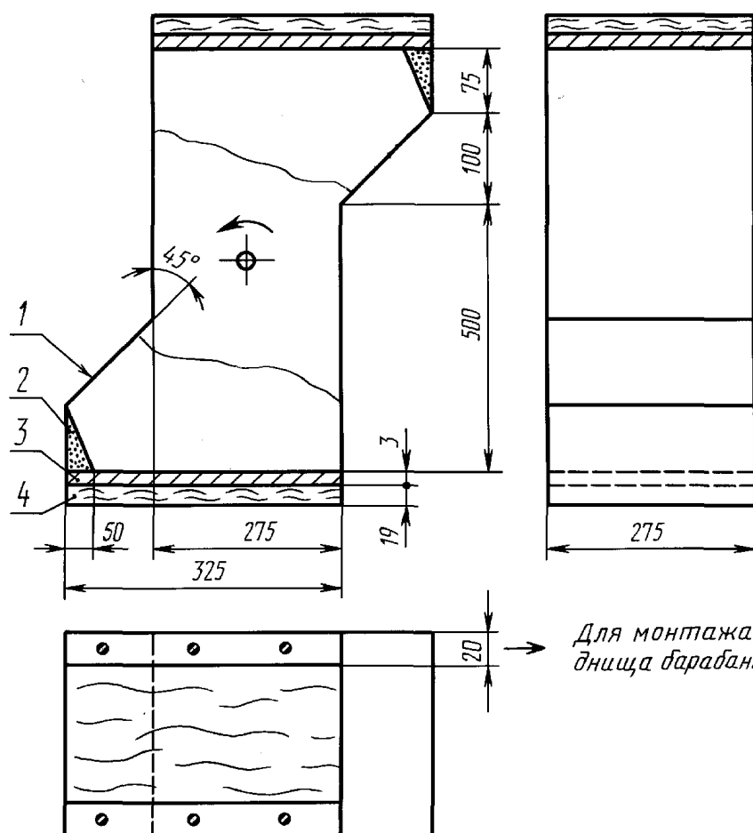
Рисунок 18 — Вращающийся барабан (ссылка — в 23.2)
