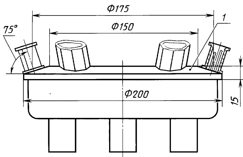
1 — стальная граненая пластинка
