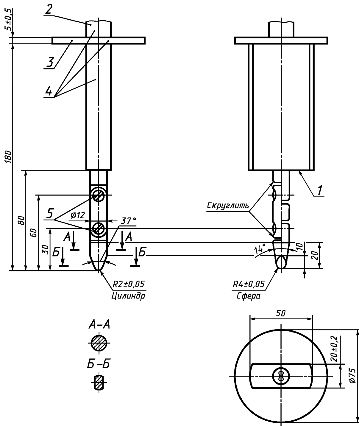
Рисунок 10 — Стандартный испытательный палец (ссылка — в 10.1)
