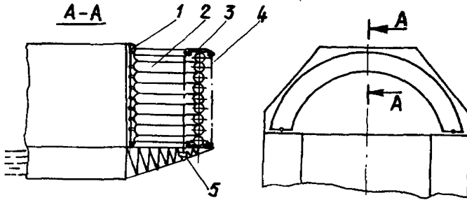
Схема ветрозащитного устройства
