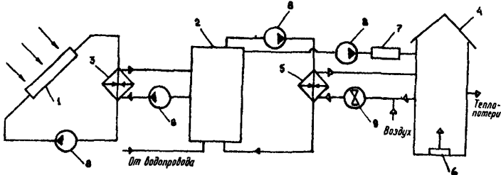
Рис.1. Принципиальная схема системы солнечного теплоснабжения
