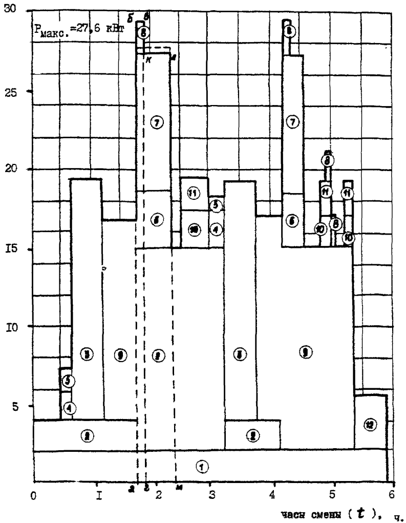
Рис.Л.4.1. Сменный график электрических нагрузок кормоцеха фермы крупного рогатого скота на 400 коров.
