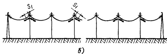
Рис.3.3. Схема установки гасителей вибрации на ВЛ:
