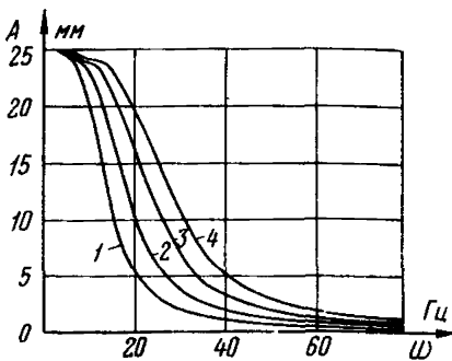
Рис.П.5. Зависимость влияния тяжения на угол вибрации провода марки АС 240/40:
