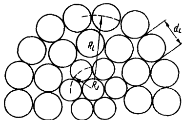
Рис. III.I. Поперечное сечение многоповивного сталеалюминиевого провода
