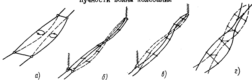
Рис. П2.2. Виды колебаний проводов, вызываемых воздействием аэродинамического следа: a - колебания проводов в подпролетах; \delta - вертикальные колебания; \theta - горизонтальные колебания; z - крутильные колебания
