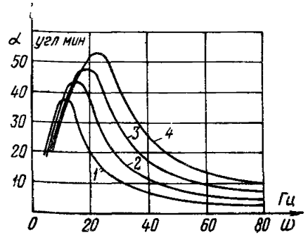
Рис.П.4. Зависимость влияния тяжения на амплитуды в пучности полуволн колебаний провода марки АС 240/40:
