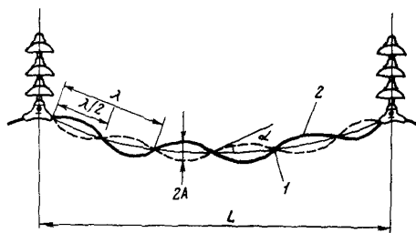
Рис.2.1. Стоячая волна вибрации провода в пролете ВЛ: I - узел колебаний; 2 - пучность; L - длина пролета; \lambda - длина волны колебаний; A - амплитуда колебаний; 2A - размах колебаний; \alpha - угол вибрации
