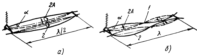
Рис. П2.1. Формы колебаний проводов в подпролетах: \alpha - с одной полуволной на подпролет; \delta - с двумя полуволнами на подпролет; I - узел колебаний; 2 - пучность колебаний; \lambda - длина волны колебаний; A - амплитуда колебаний; \alpha - угол колебаний в подпролетах; \Theta - траектория движения провода в пучности волны колебаний
