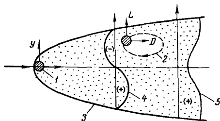
Рис. П2.3. Аэродинамические силы, действующие на подветренный провод: L - подъемная сила; D - сила лобового сопротивления; 1 - наветренный провод; 2 - траектория движения подветренного провода; 3 - граница аэродинамического следа; 4 - эпюра подъемной силы в сечении следа; 5 - эпюра лобового сопротивления в сечении следа
