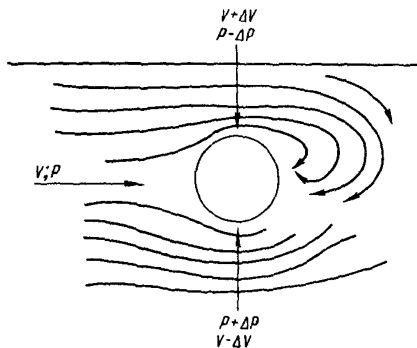
Рис.2.3. Схема вихреобразования за проводом
