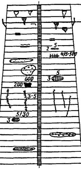
Образец карты дефектов железобетонной дымовой трубы и таблицы прочности бетона ее ствола
