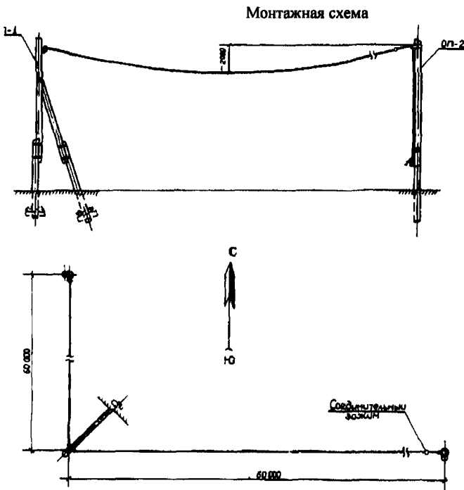
Рис.6. Рабочий чертёж гололедного поста, выполненный Украинским отделением института «Сельэнергопроект»
