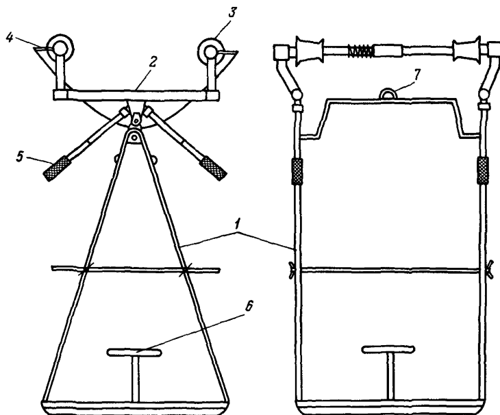
Рис.7. Универсальное монтерское сиденье-тележка:
