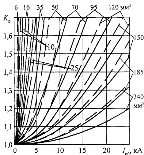
Рис. 6.8. Зависимости коэффициента увеличения активного сопротивления кабелей различных сечений с алюминиевыми жилами от тока дугового устойчивого КЗ с учетом теплоотдачи при продолжительностях КЗ 0,2 с (сплошные кривые) и 0,6 с (пунктирные кривые)
