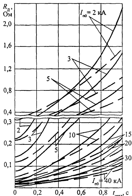
Рис. 5.18. Зависимость R_d = f(t_{откл}, I_{но}) при КЗ в электроустановках с кабельными линиями напряжением 6 кВ (сплошные кривые) и 10 кВ (пунктирные кривые)
