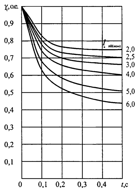
Рис. 5.4. Типовые кривые изменения периодической составляющей тока КЗ от турбогенераторов типов ТВВ-1000-2У3 и ТВВ-1200-2У3 с диодной бесщеточной системой возбуждения
