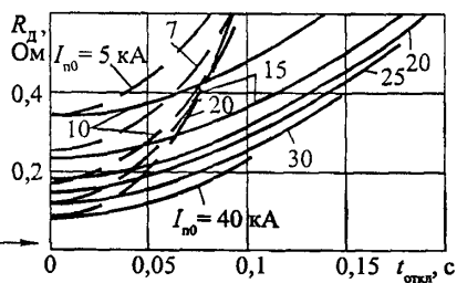
Рис. 5.19. Зависимость R_d = f(t_{откл}, I_{но}) при КЗ на воздушных линиях 35 кВ (сплошные кривые) и 10 кВ (пунктирные кривые)
