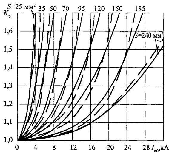
Рис. 5.23. Зависимость K_\theta = f(I_{\text{н}}, S_{\text{кб}}) для кабелей с алюминиевыми жилами с учетом теплоотдачи и сопротивления дуги
