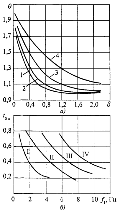
Рис. 7.9. К определению коэффициента превышения \theta в зависимости от \delta , t_{\text{бн}} , f_1
