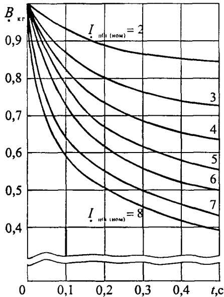
Рис. 8.2. Кривые для определения B_{kr} от синхронных генераторов с тиристорной системой возбуждения
