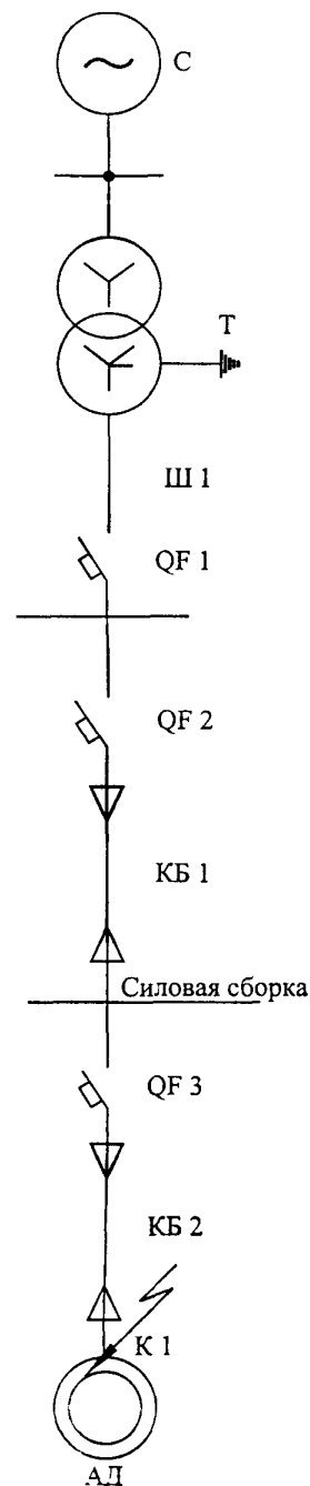
Рис. 6.12. Расчетная схема к примеру 6.11.1
