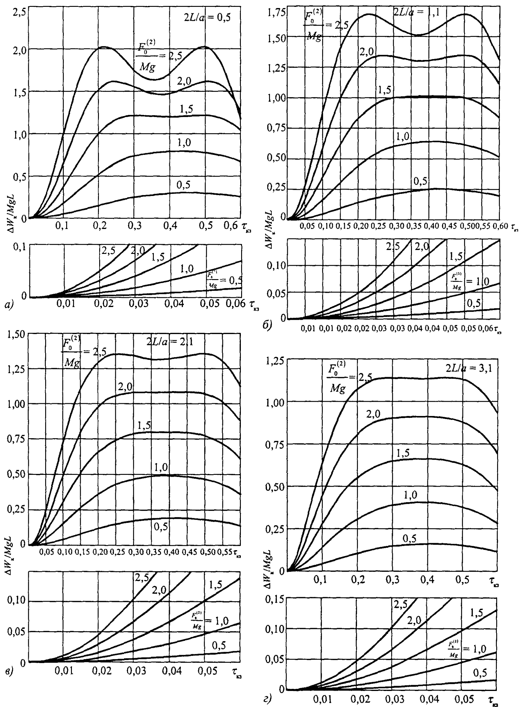
Рис. 7.11. Характеристики \Delta W^*/MgL при двухфазном КЗ (см. также с. 118)
