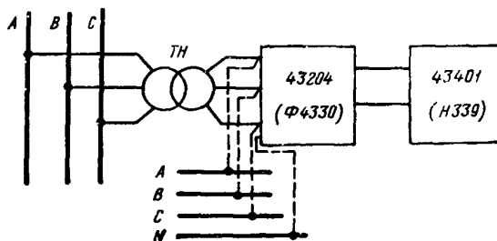
Рис.8.16. Схема измерения коэффициентов обратной и нулевой последовательностей напряжения с помощью приборов 43204 и 43401 или Ф4330 и НЗ39 (43401)
