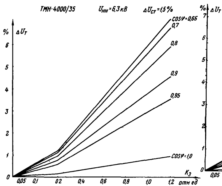
Рис. III.19. Графики потерь напряжения в трансформаторе 35/6 кВ мощностью 4000 кВ·А
