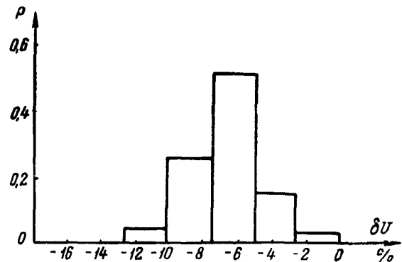
Рис.10.2. Гистограмма отклонения напряжения, построенная на основе регистрограммы
