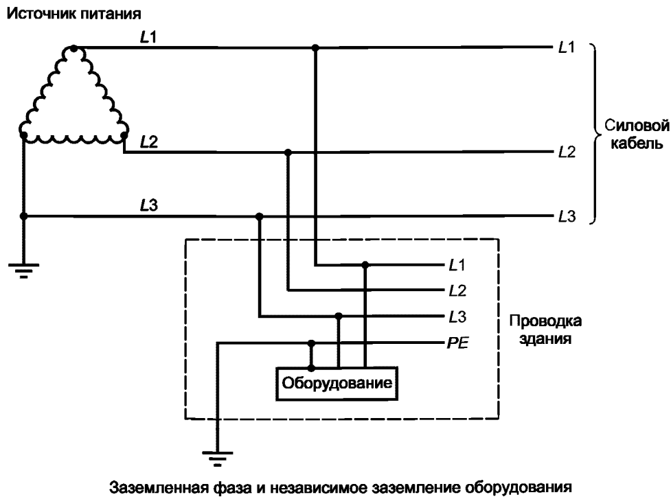
Рисунок V.6 — Пример трехпроводной ТТ системы энергоснабжения
