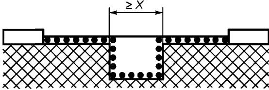
Рисунок F.1 — Узкая канавка Условные обозначения к рисункам F.1—F.13 ———— - ЗАЗОР; ..... - ПУТЬ УТЕЧКИ.
