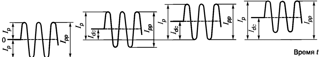
Рисунок М.3 — Амплитуда и размах амплитуд тока
