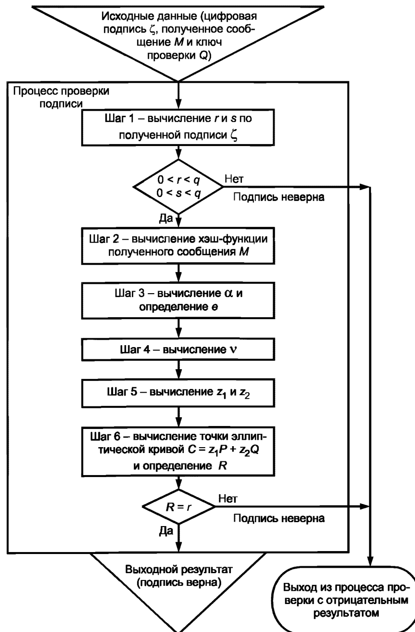
Рисунок 3 — Схема процесса проверки цифровой подписи
