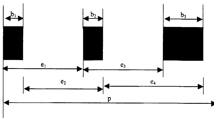
Рисунок 5 — Декодирование размеров
