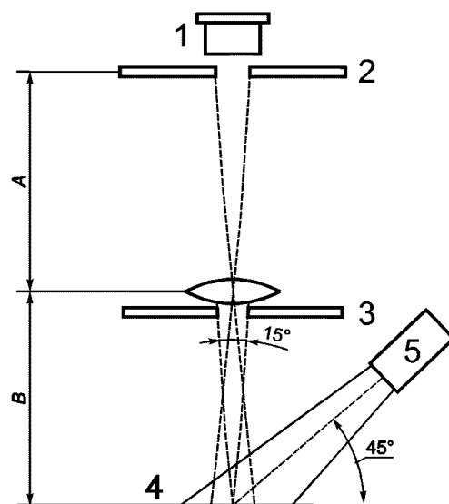
1 — фотоувеличительный элемент; 2 — апертура при линейном увеличении 1:1 (размер A равен размеру B ); 3 — диафрагма; 4 — образец; 5 — источник оптического излучения
