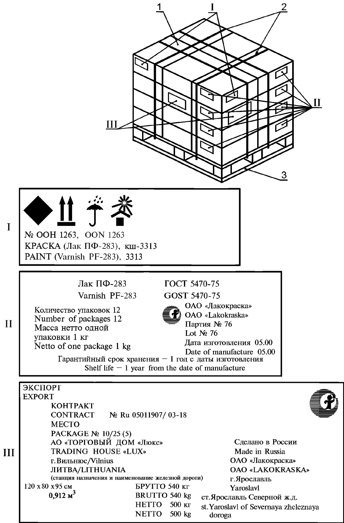
I и III — транспортная маркировка; II — маркировка, характеризующая продукцию; 1 — ящик, 2 — лента, 3 — поддон Рисунок К.2 — Маркировка продукции в картонных ящиках, сформированных в транспортный пакет
