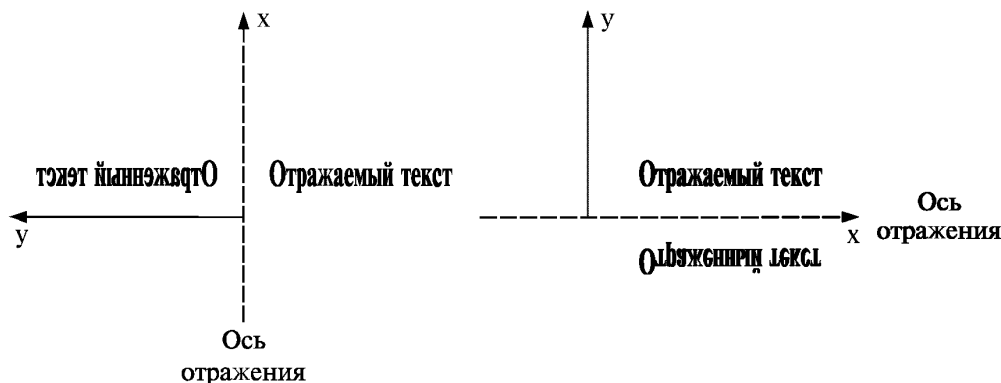
Рисунок 24 — Стиль текста с зеркальным отображением
