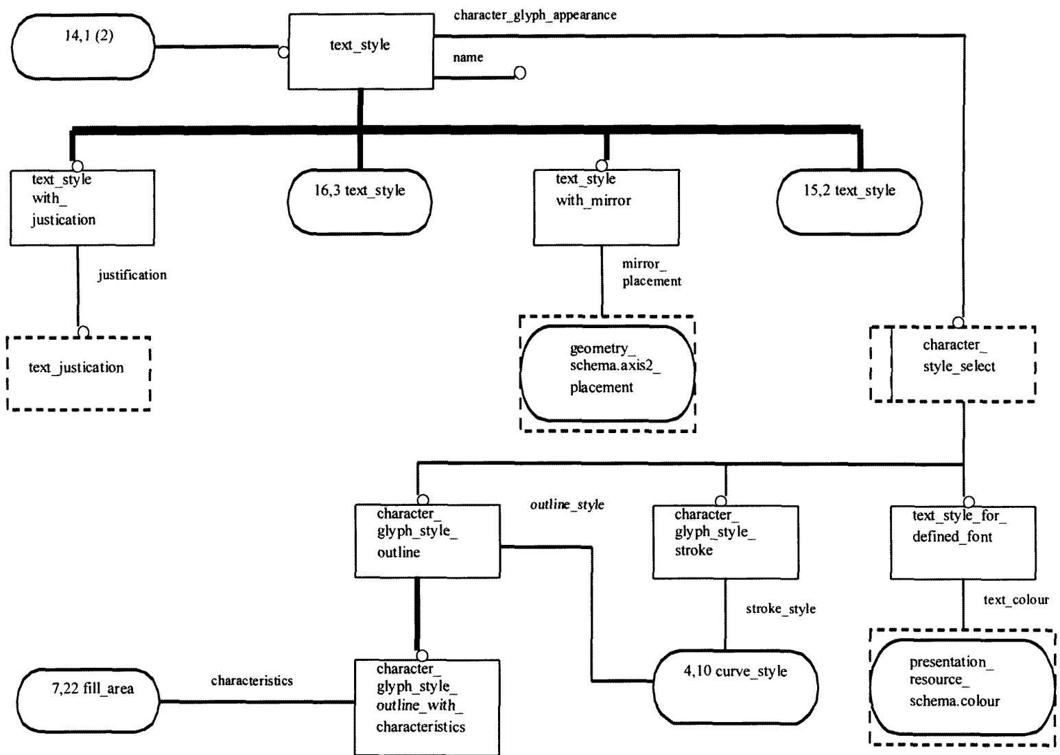
Рисунок Е.30 — EXPRESS-G диаграмма presentation_appearance_schema 14 из 21
