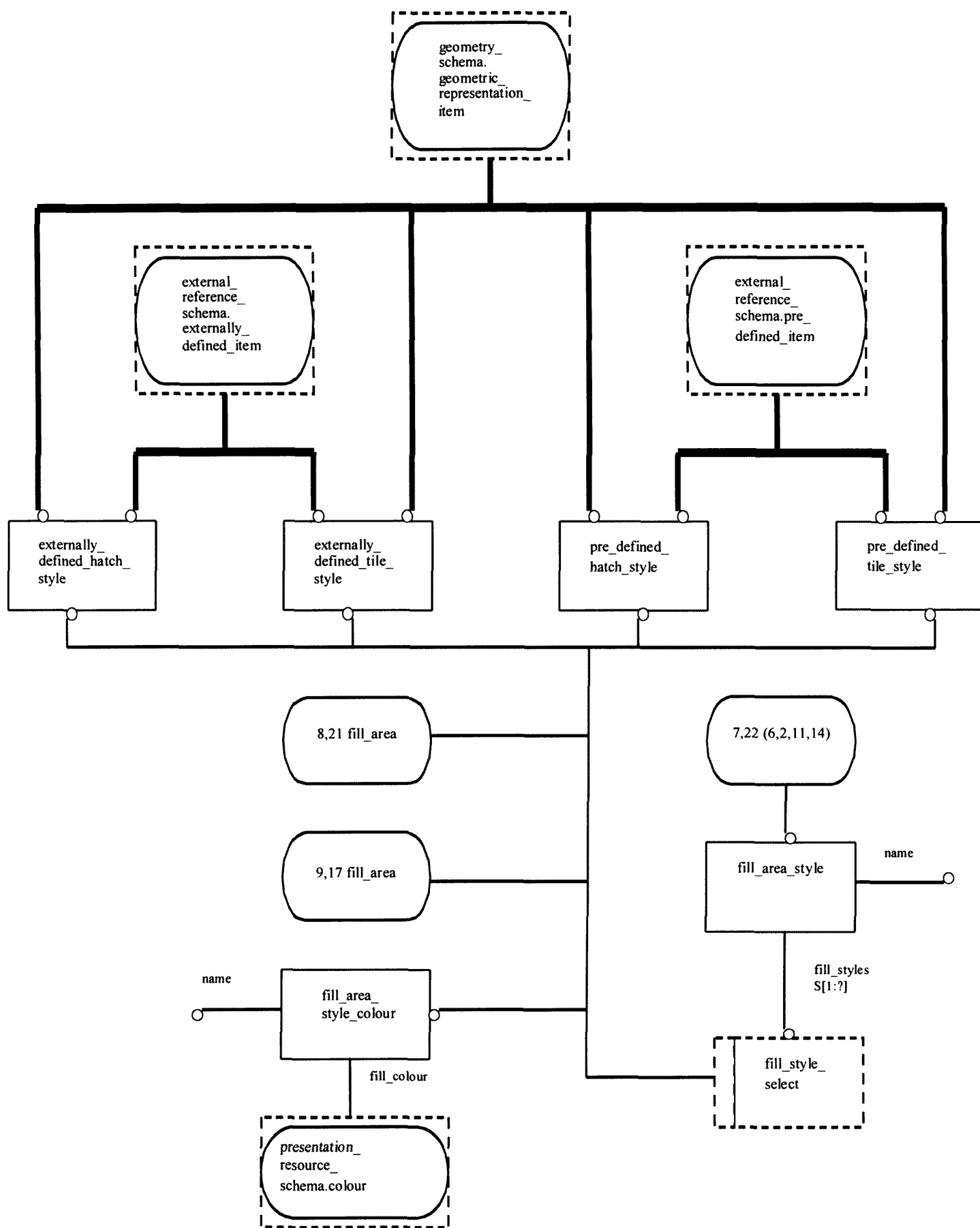
Рисунок Е.23 — EXPRESS-G диаграмма presentation_appearance_schema 7 из 21
