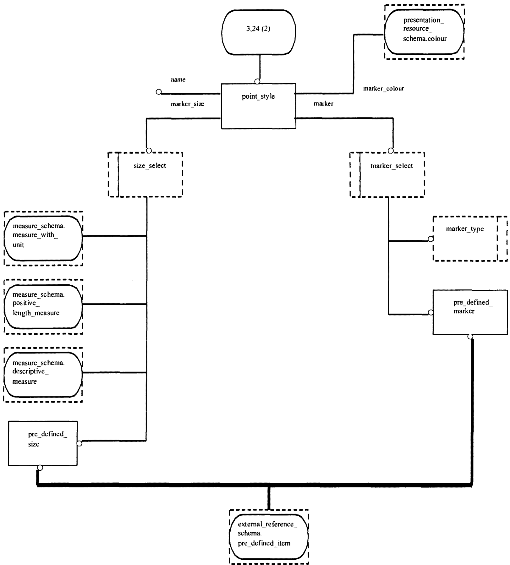
Рисунок Е.19 — EXPRESS-G диаграмма presentation_appearance_schema 3 из 21
