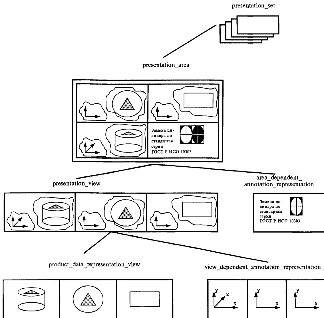
Рисунок 2 — Пример иерархии представления
