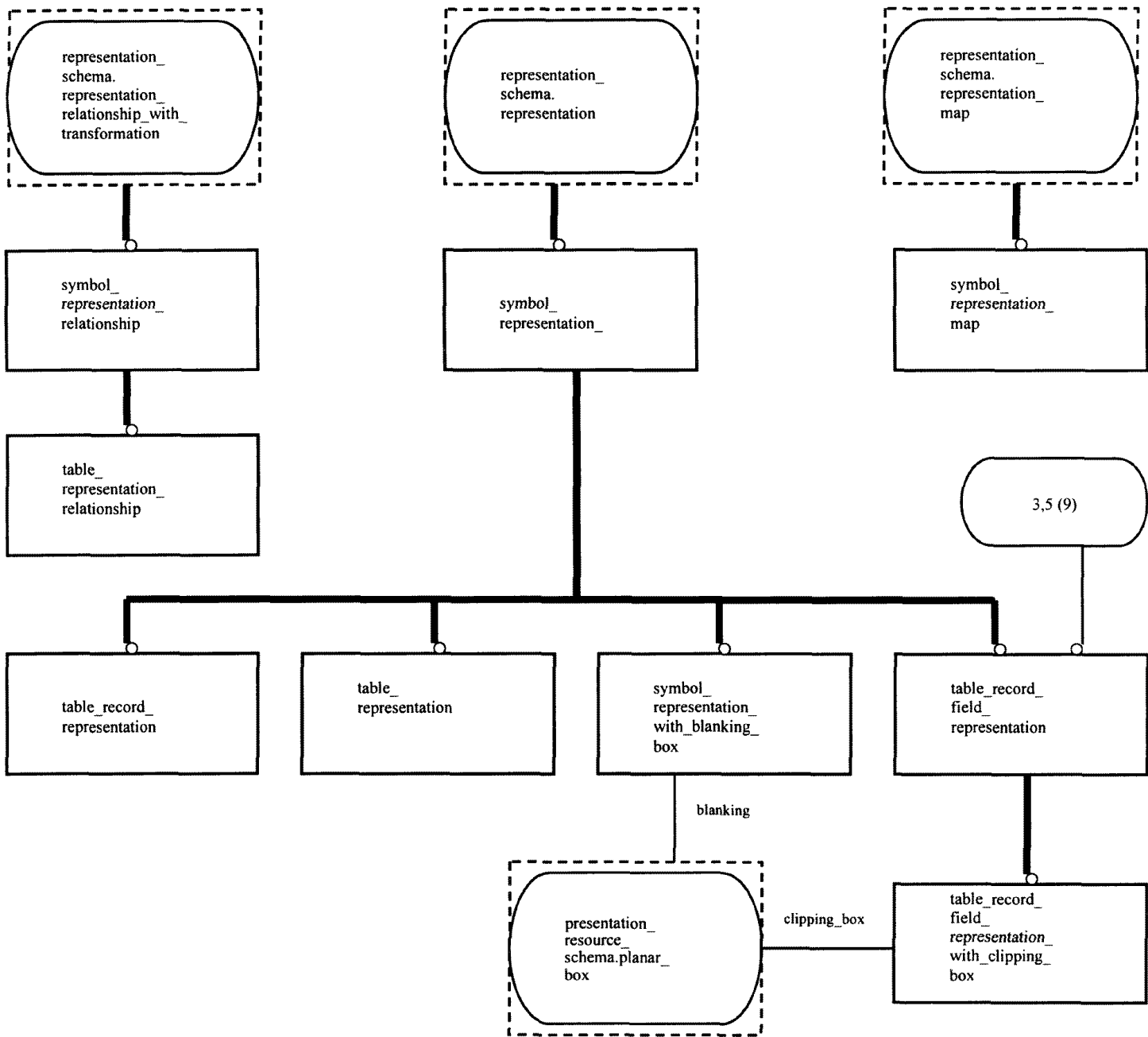
Рисунок Е.10 — EXPRESS-G диаграмма presentation_definition_schema 3 из 9
