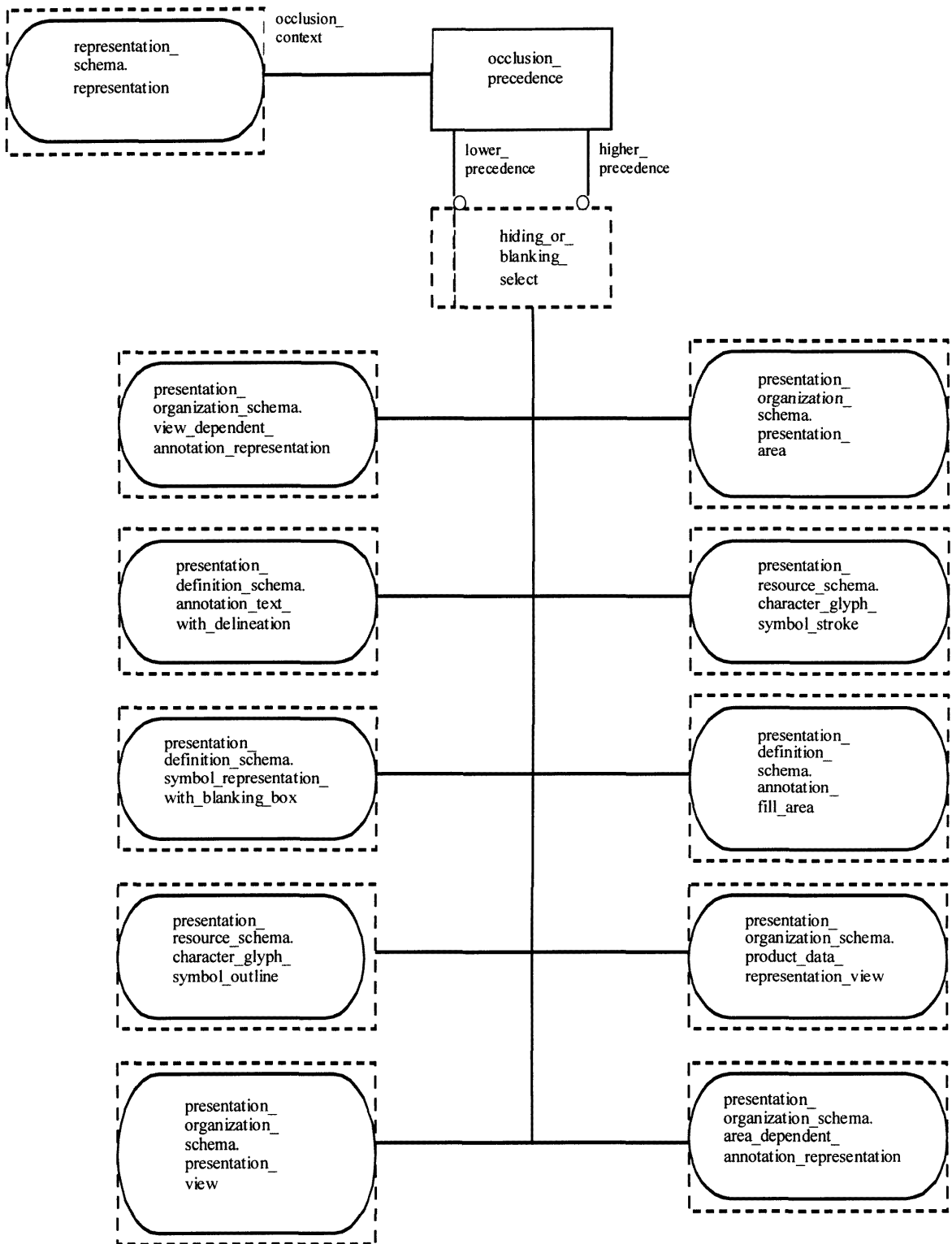
Рисунок Е.36 — EXPRESS-G диаграмма presentation_appearance_schema 20 из 21
