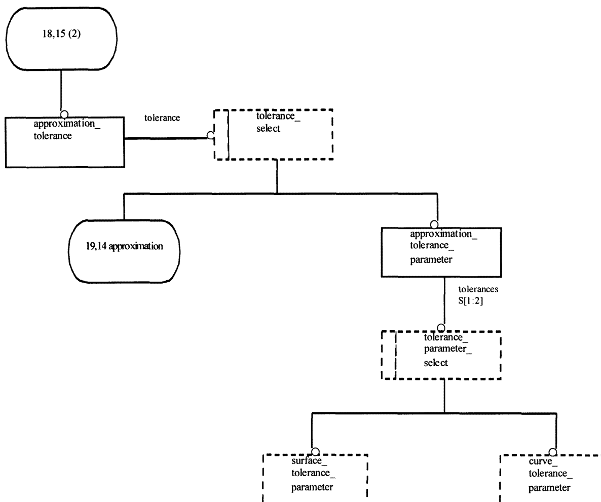
Рисунок Е.34 — EXPRESS-G диаграмма presentation_appearance_schema 18 из 21
