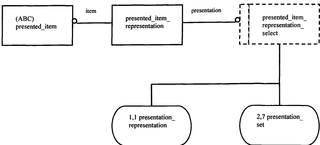
Рисунок Е.7 — EXPRESS-G диаграмма presentation_organization_schema 7 из 7
