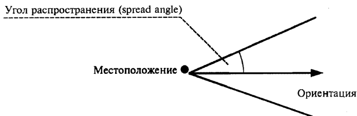
Рисунок 11 — Распространение потока от источника света (объект light_source_spot )
