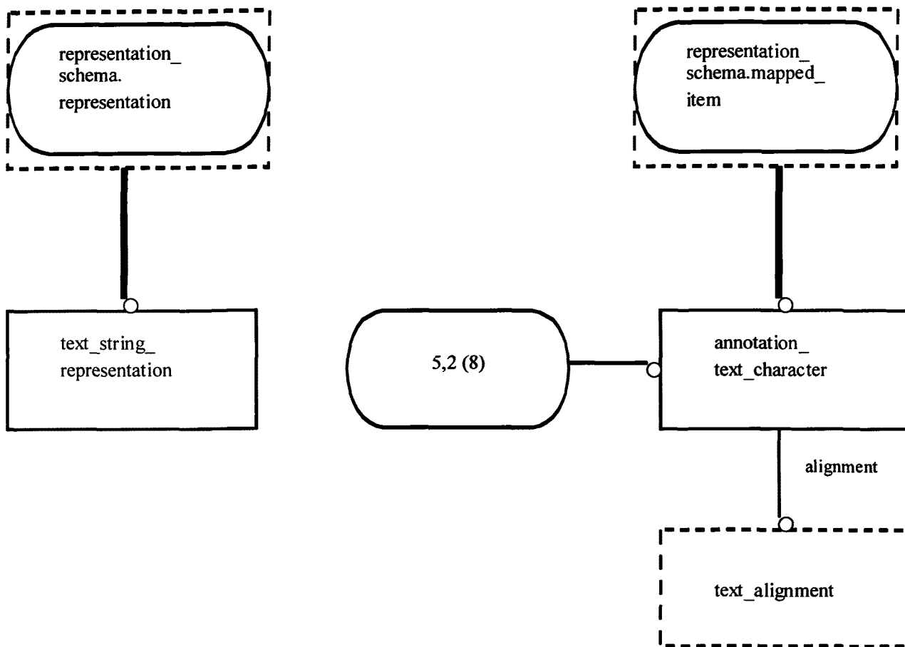
Рисунок Е.12 — EXPRESS-G диаграмма presentation_definition_schema 5 из 9
