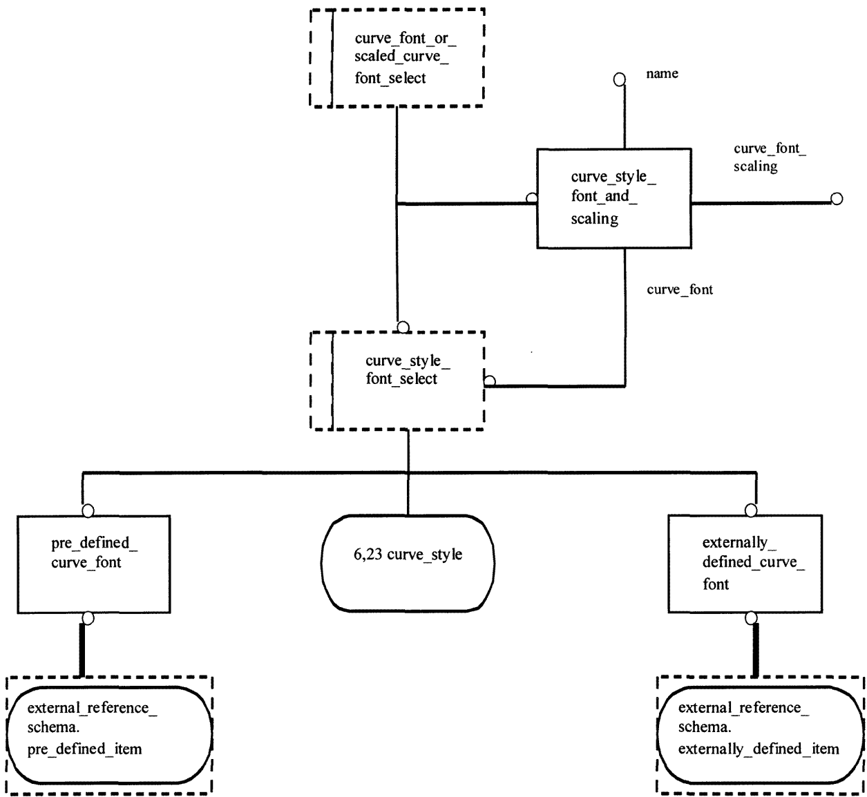
Рисунок Е.21 — EXPRESS-G диаграмма presentation_appearance_schema 5 из 21
