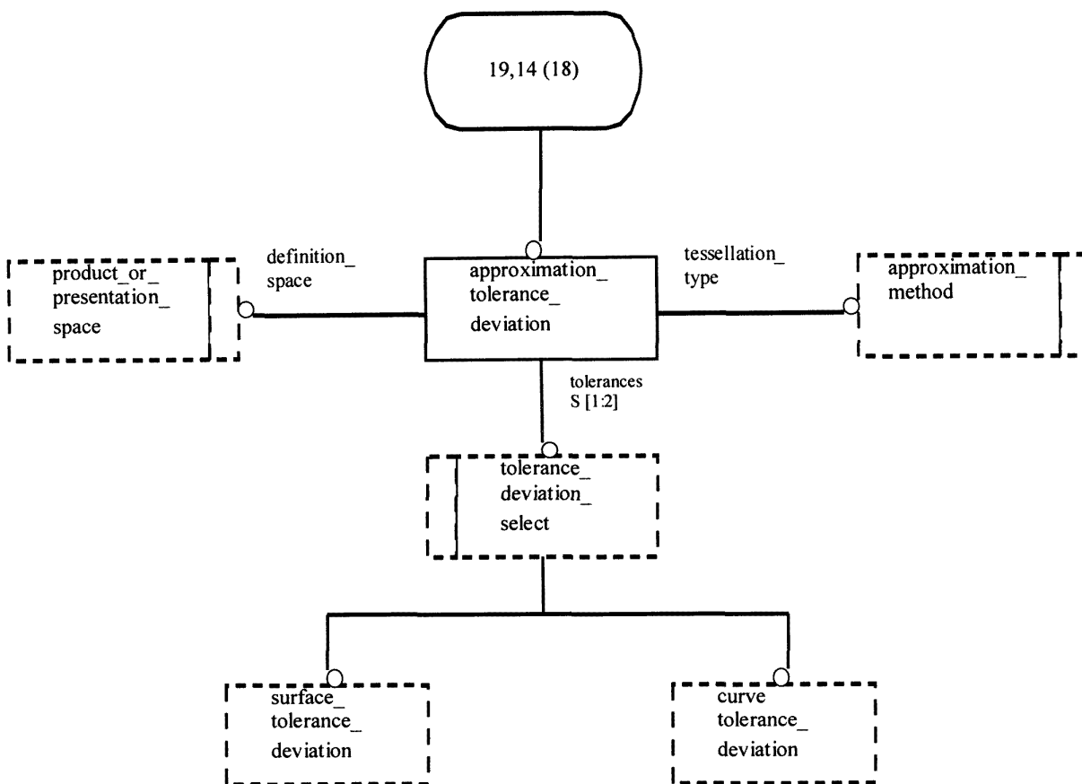
Рисунок Е.35 — EXPRESS-G диаграмма presentation_appearance_schema 19 из 21
