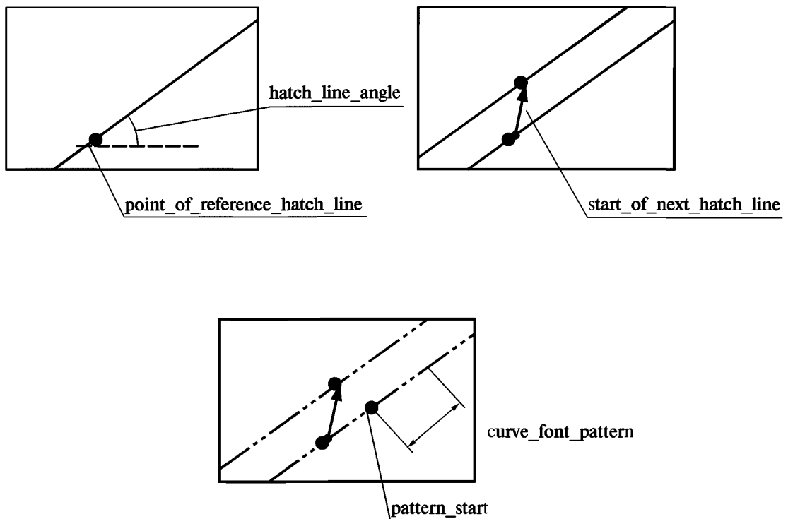
Рисунок 21 — Стиль штриховки зашиваемой области
