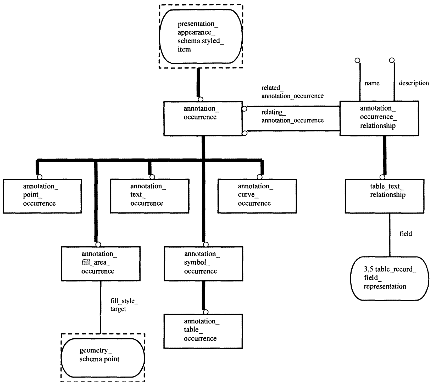
Рисунок E.16 — EXPRESS-G диаграмма presentation_definition_schema 9 из 9
