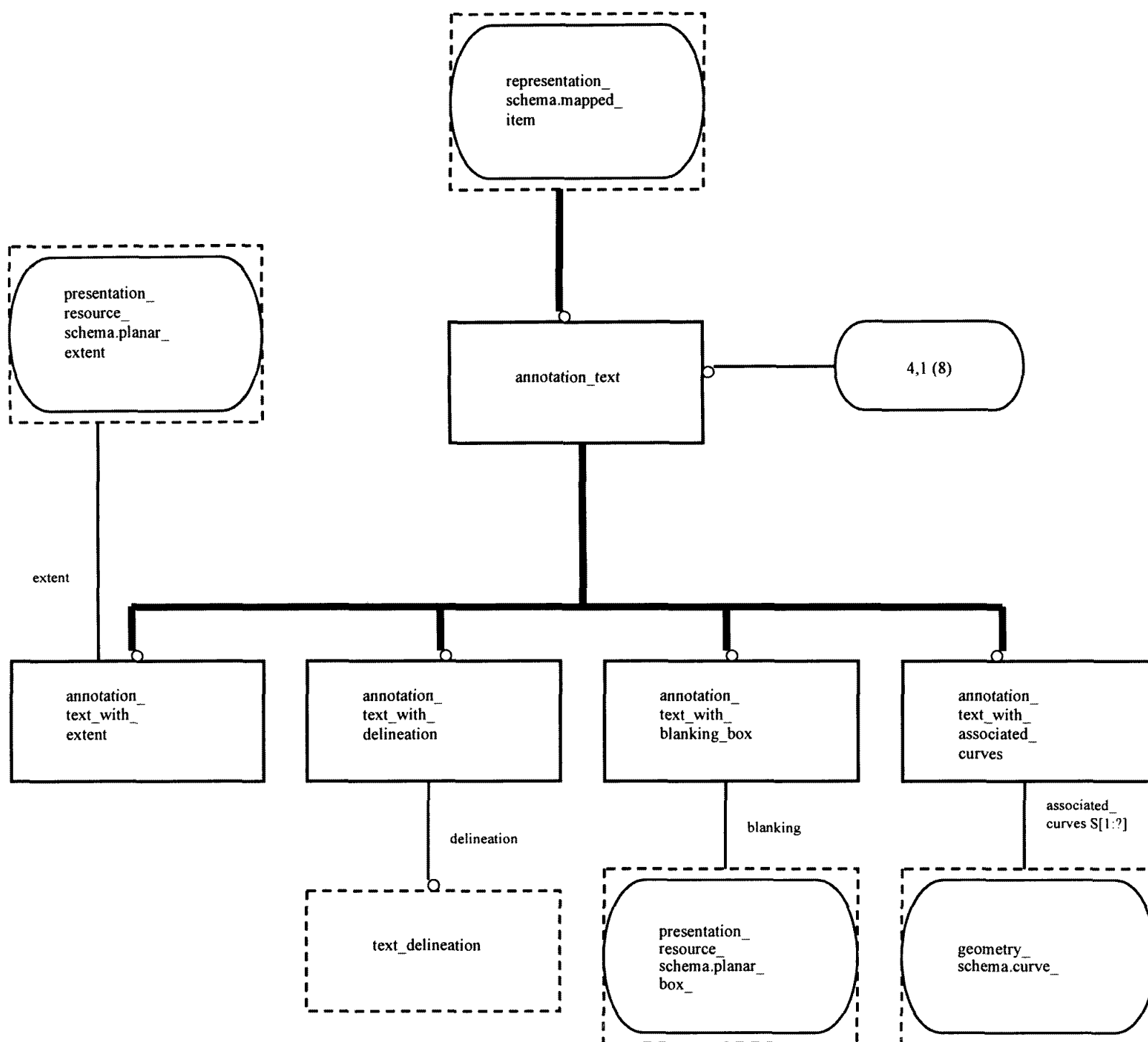
Рисунок Е.11 — EXPRESS-G диаграмма presentation_definition_schema 4 из 9
