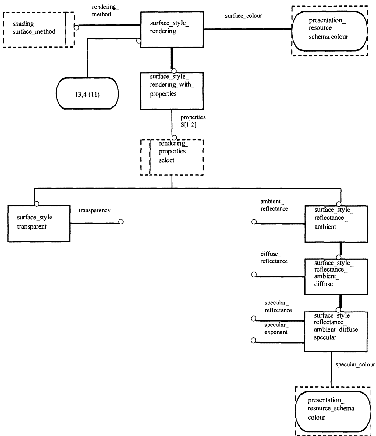
Рисунок Е.29 — EXPRESS-G диаграмма presentation_appearance_schema 13 из 21
