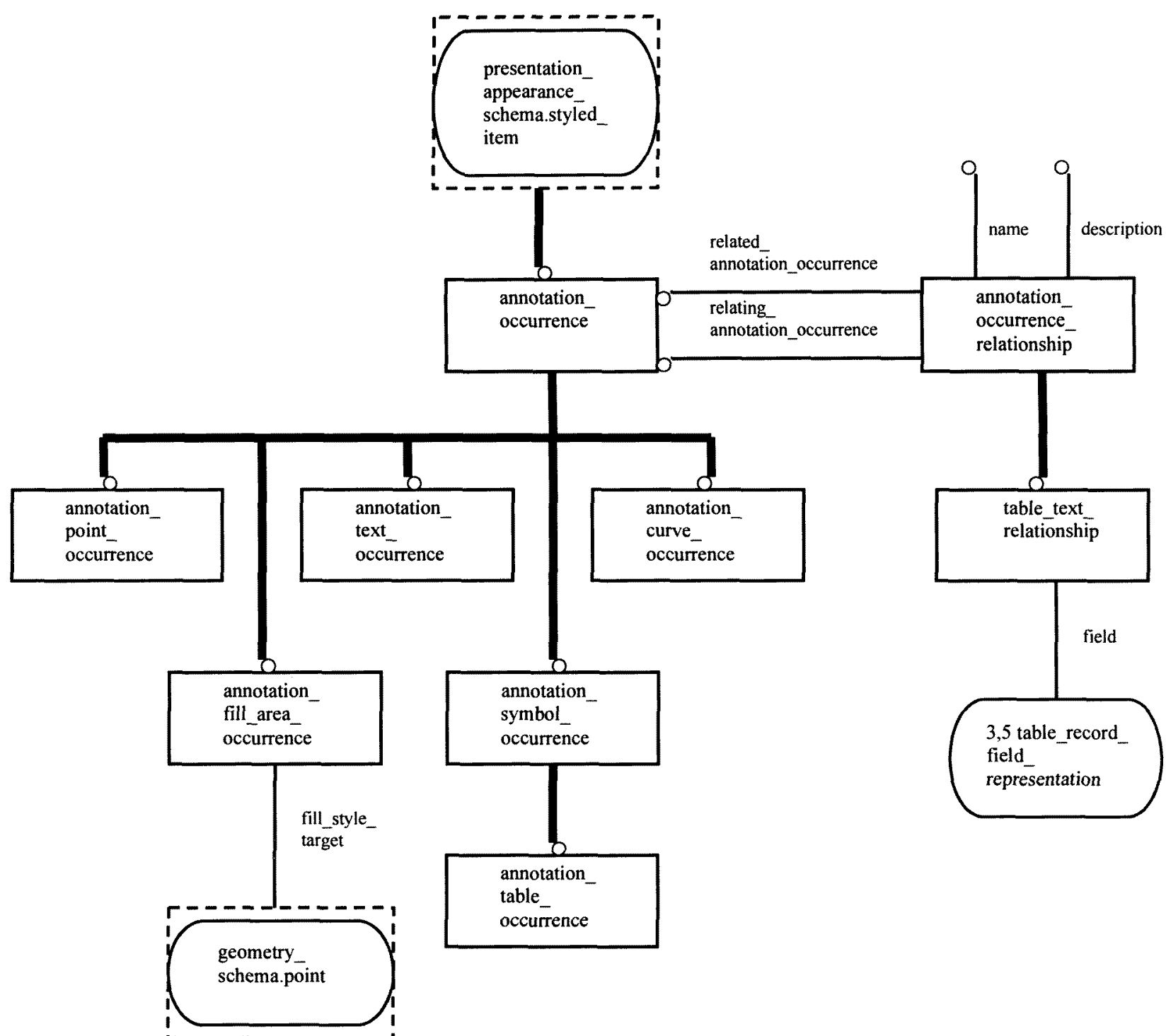
Рисунок Е.16 — EXPRESS-G диаграмма presentation_definition_schema 9 из 9
