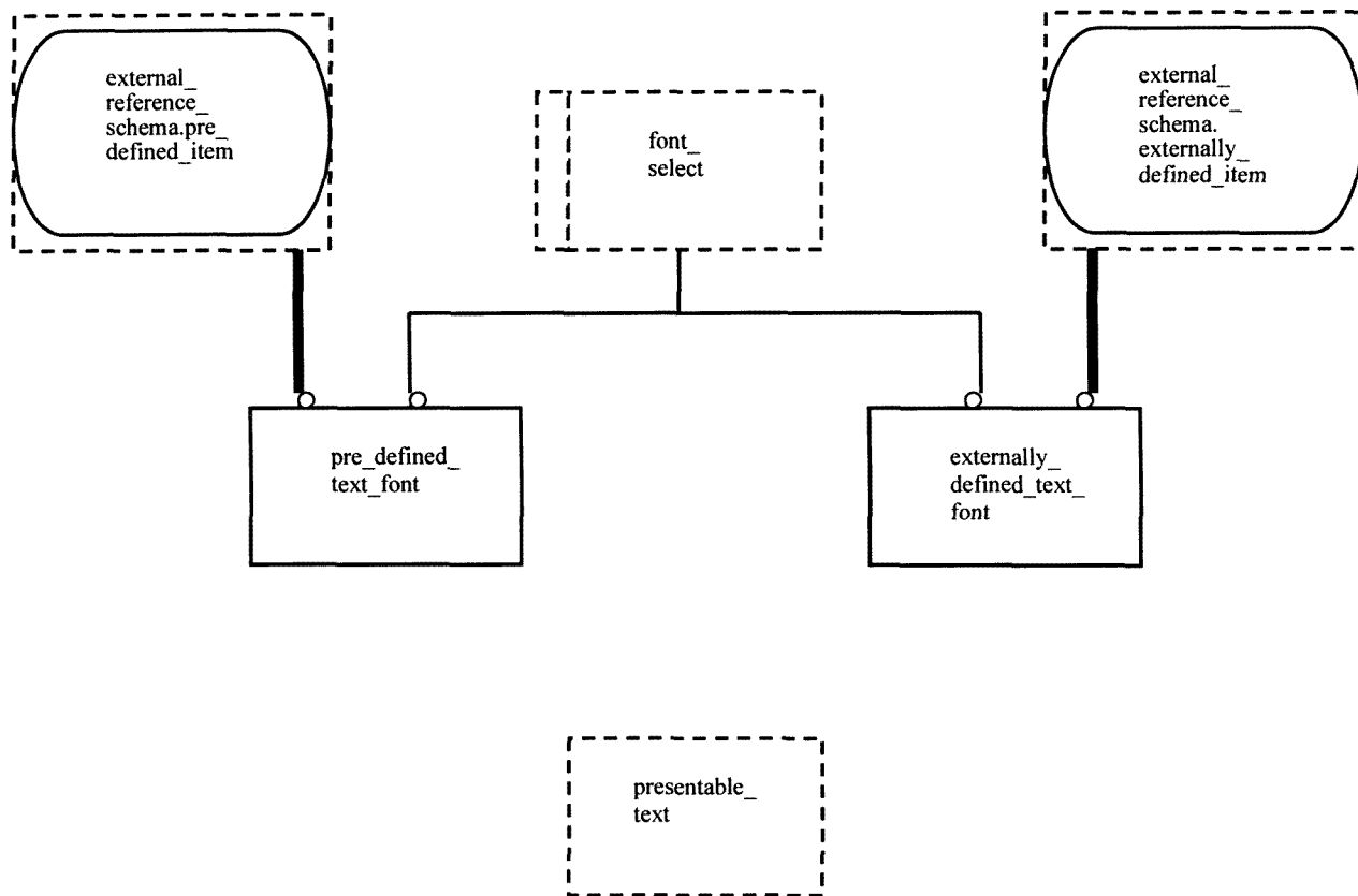
Рисунок Е.40 — EXPRESS-G диаграмма presentation_resource_schema 3 из 5
