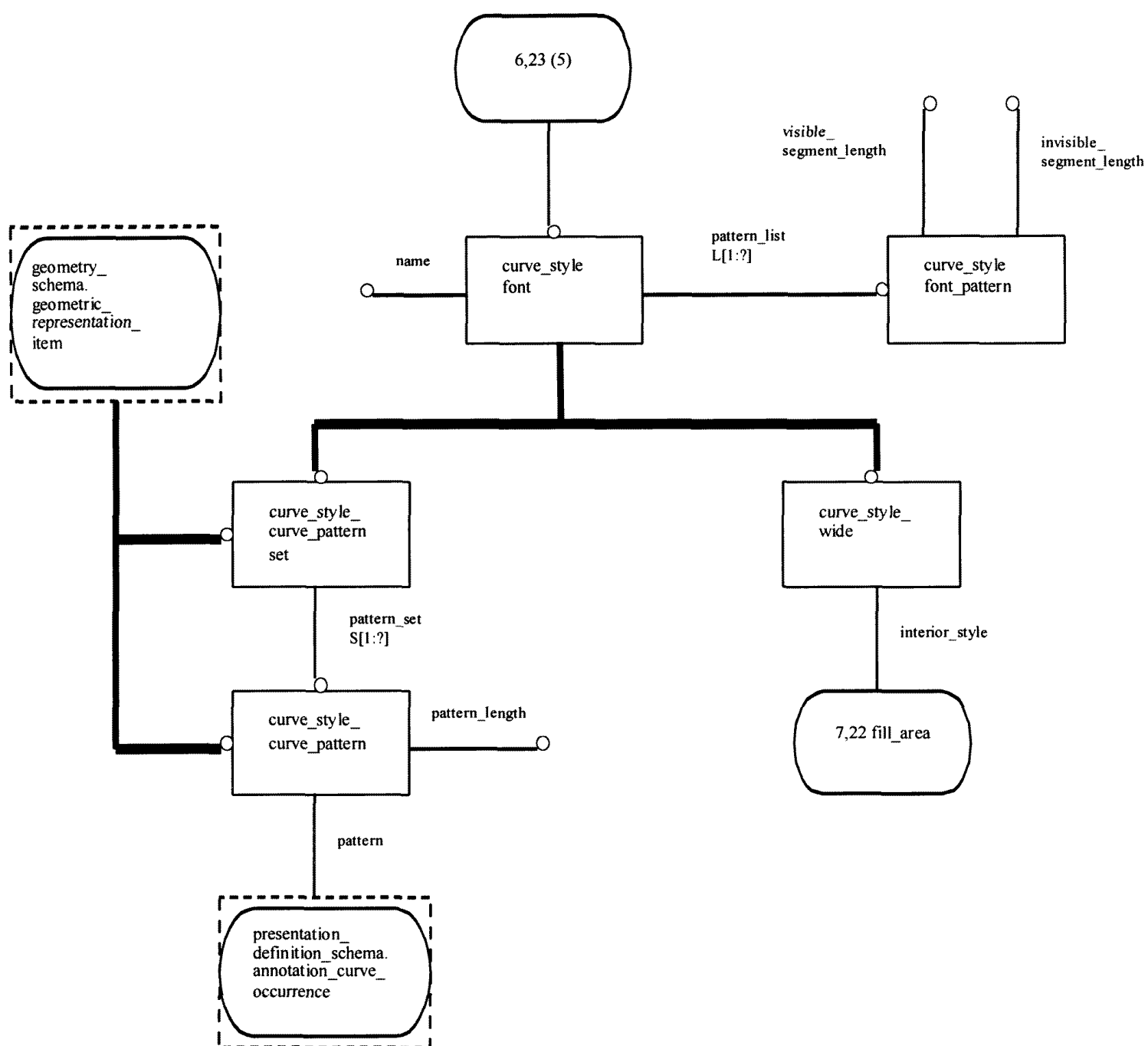
Рисунок Е.22 — EXPRESS-G диаграмма presentation_appearance_schema 6 из 21
