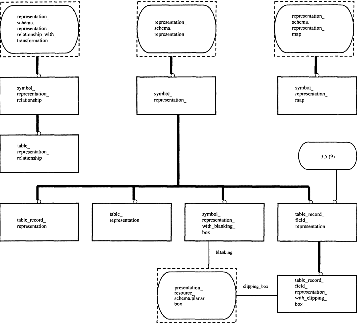
Рисунок Е.10 — EXPRESS-G диаграмма presentation_definition_schema 3 из 9
