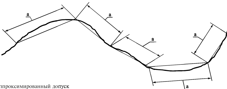
Рисунок 18 — Отклонение и длина хорды
