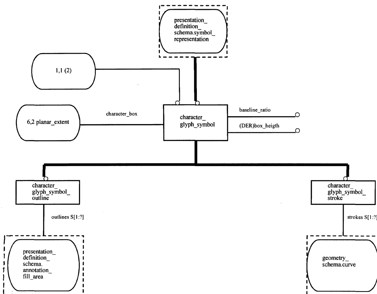
Рисунок Е.38 — EXPRESS-G диаграмма presentation_resource_schema 1 из 5
