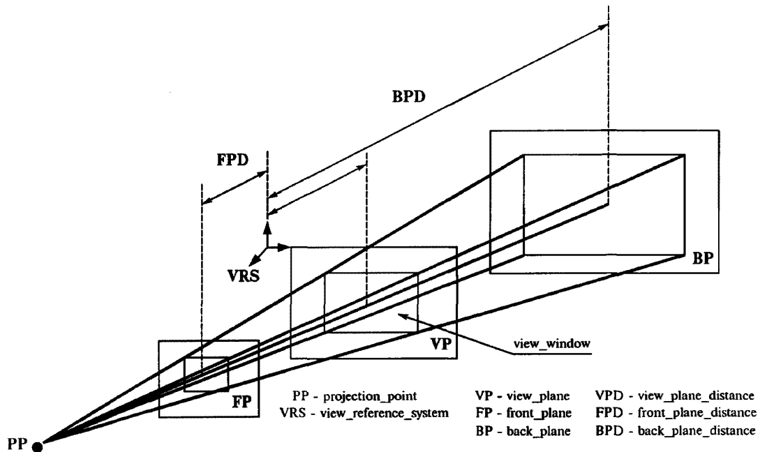
Рисунок 7 — Вид объема, тип проекции — CENTRAL
