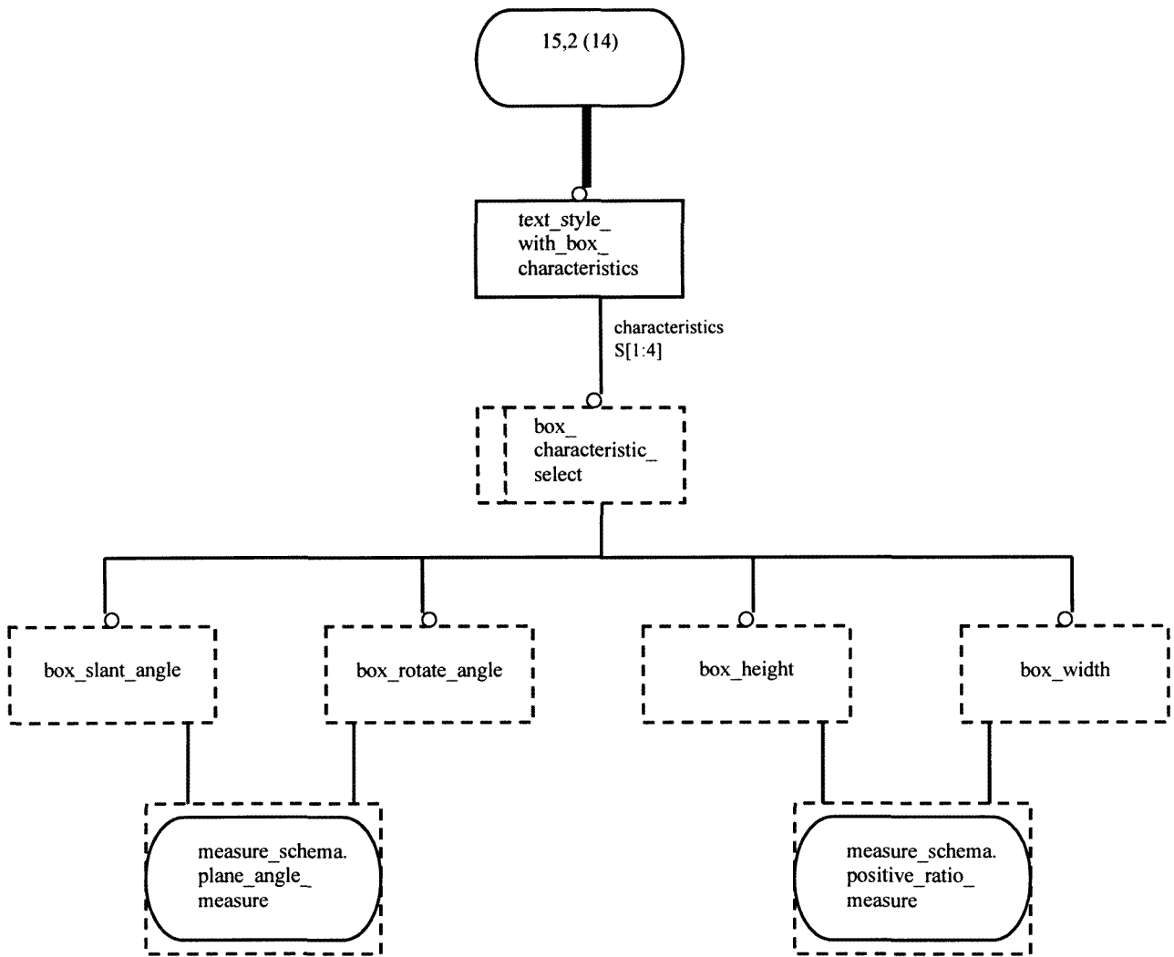
Рисунок Е.31 — EXPRESS-G диаграмма presentation_appearance_schema 15 из 21
