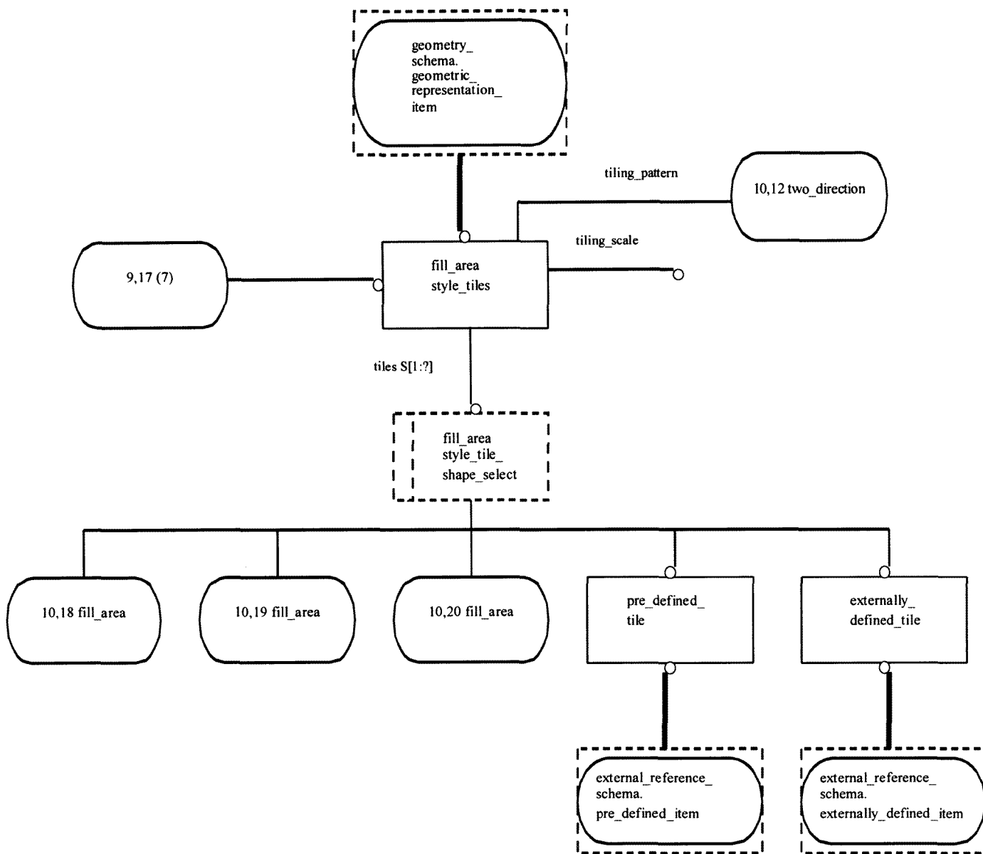
Рисунок E.25 — EXPRESS-G диаграмма presentation_appearance_schema 9 из 21
