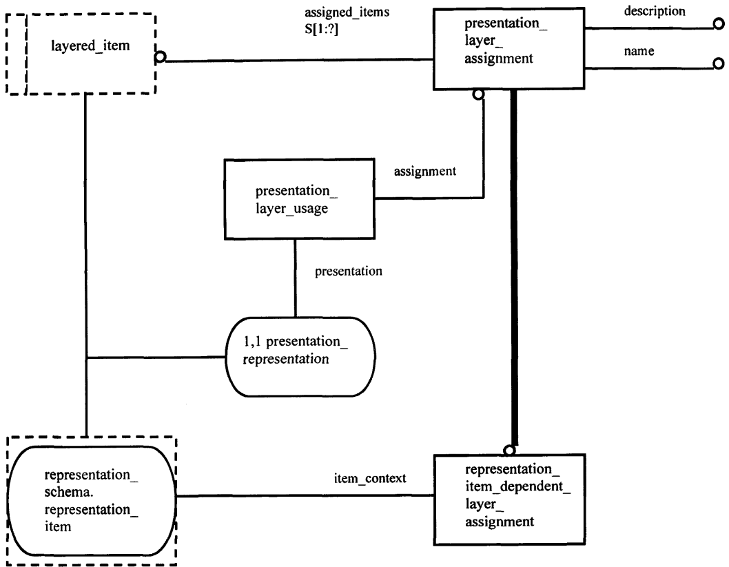
Рисунок Е.6 — EXPRESS-G диаграмма presentation_organization_schema 6 из 7
