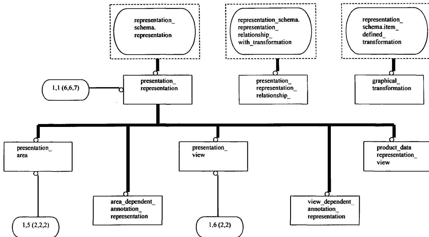
Рисунок Е.1 — EXPRESS-G диаграмма presentation_organization_schema 1 из 7
