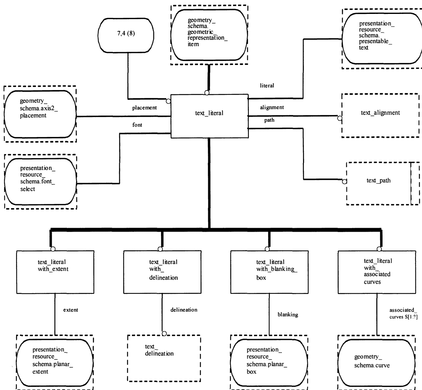
Рисунок E.14 — EXPRESS-G диаграмма presentation_definition_schema 7 из 9
