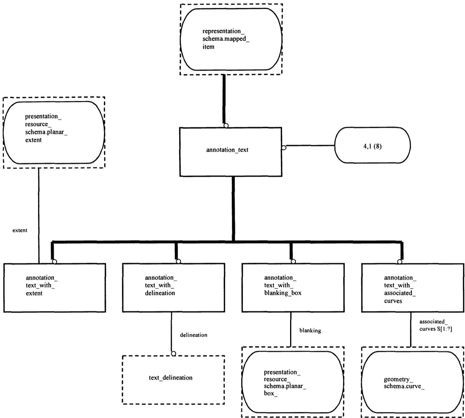
Рисунок E.11 — EXPRESS-G диаграмма presentation_definition_schema 4 из 9
