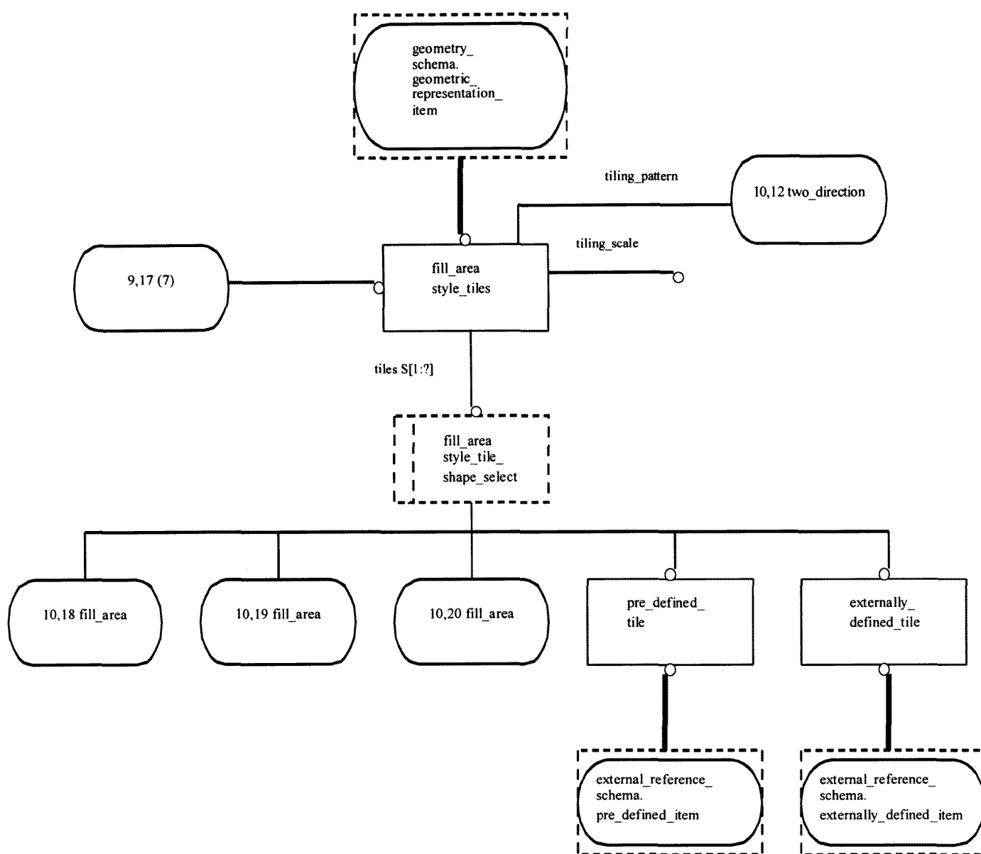
Рисунок Е.25 — EXPRESS-G диаграмма presentation_appearance_schema 9 из 21
