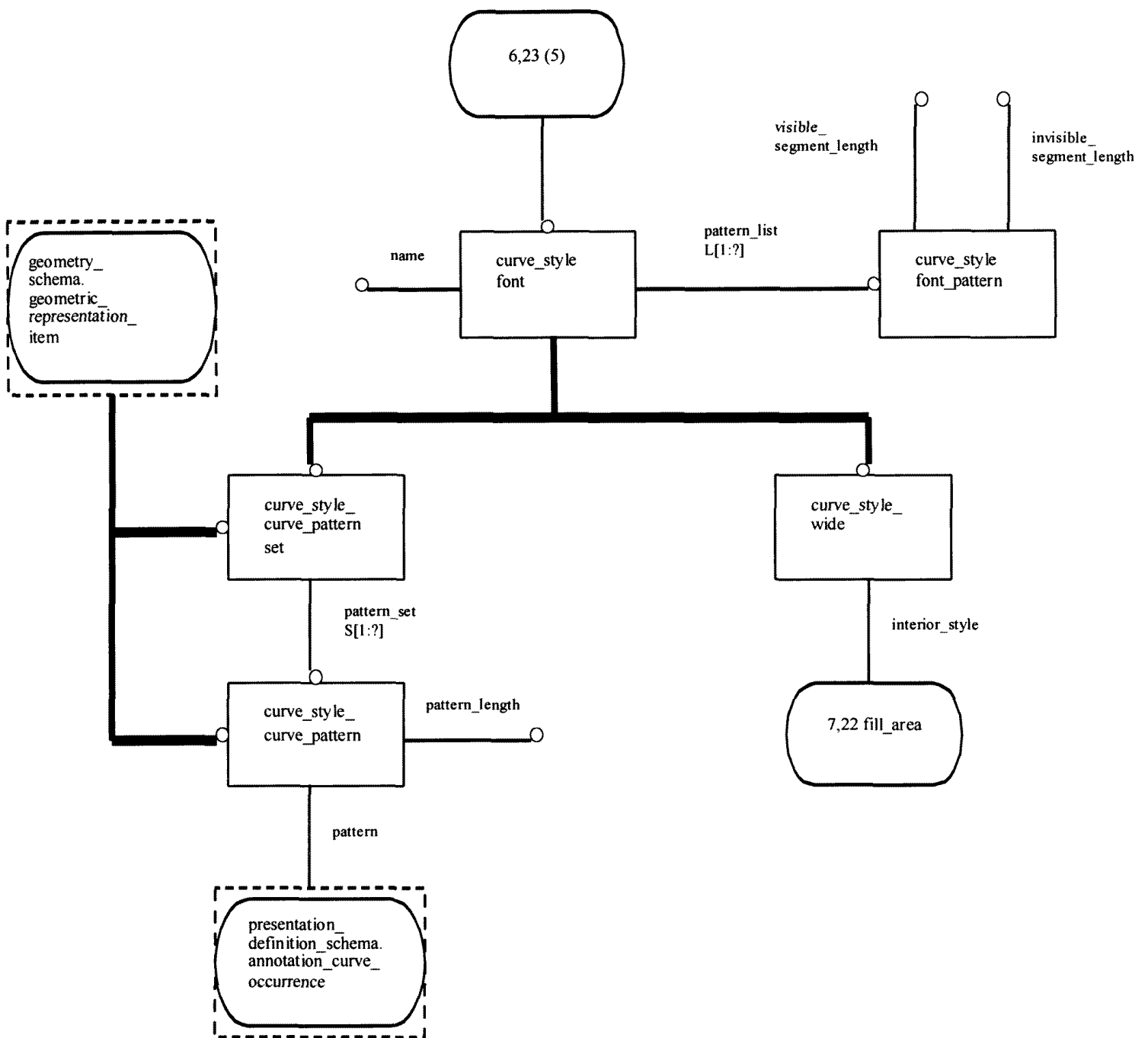
Рисунок E.22 — EXPRESS-G диаграмма presentation_appearance_schema 6 из 21
