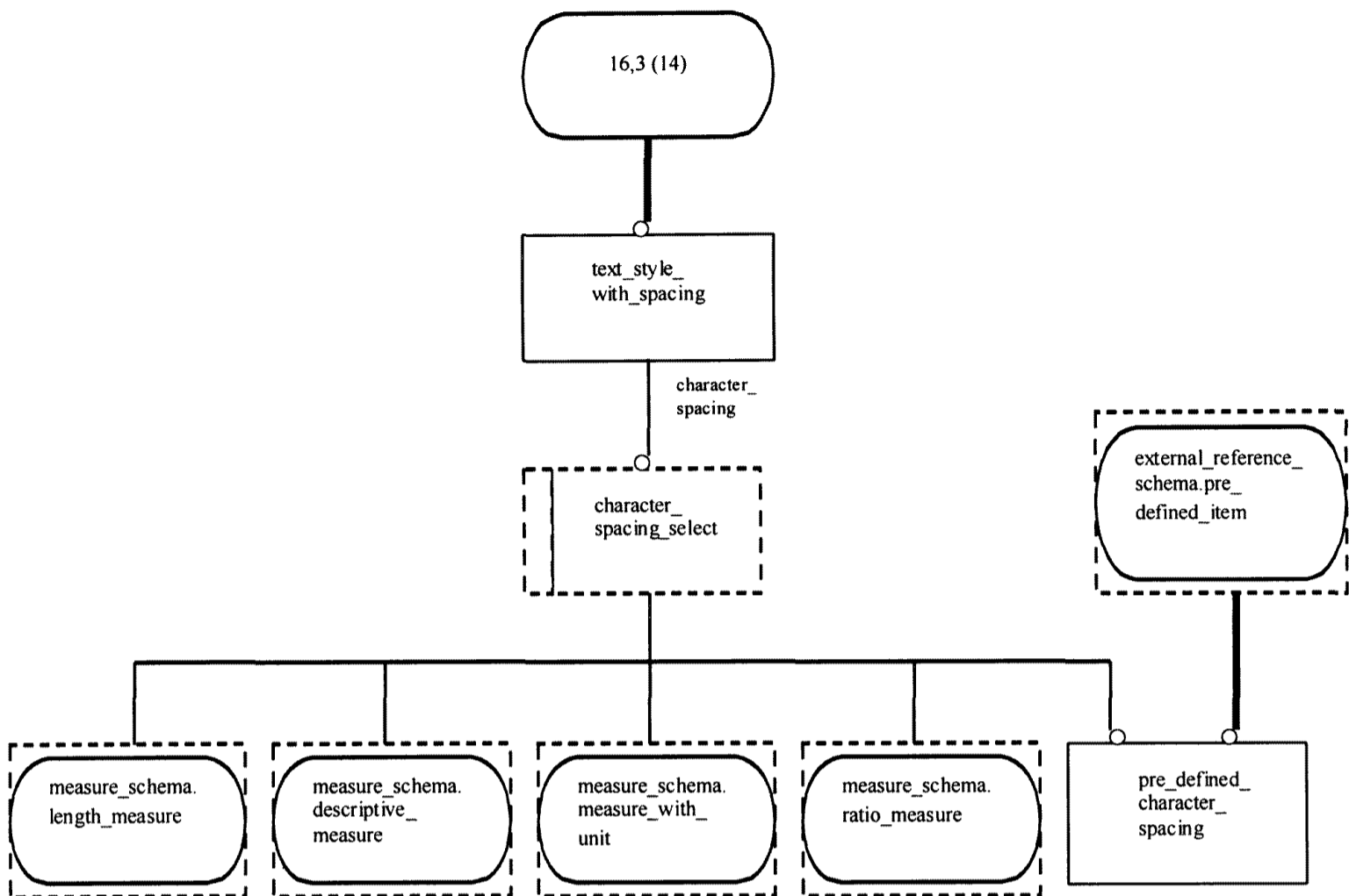
Рисунок Е.32 — EXPRESS-G диаграмма presentation_appearance_schema 16 из 21
