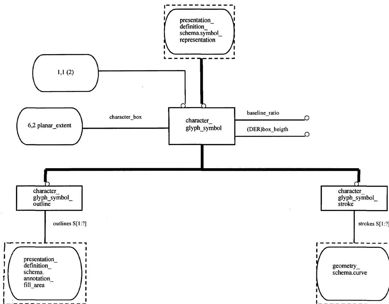
Рисунок E.38 — EXPRESS-G диаграмма presentation_resource_schema 1 из 5
