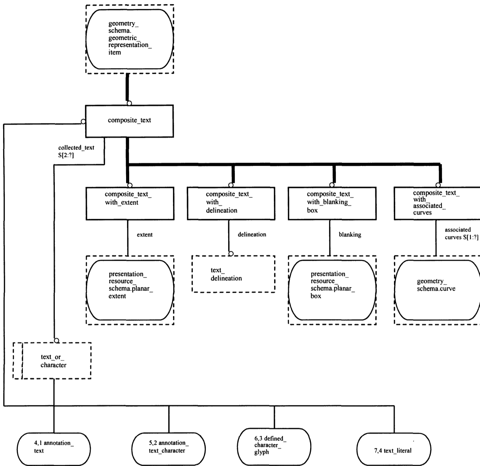
Рисунок Е.15 — EXPRESS-G диаграмма presentation_definition_schema 8 из 9
