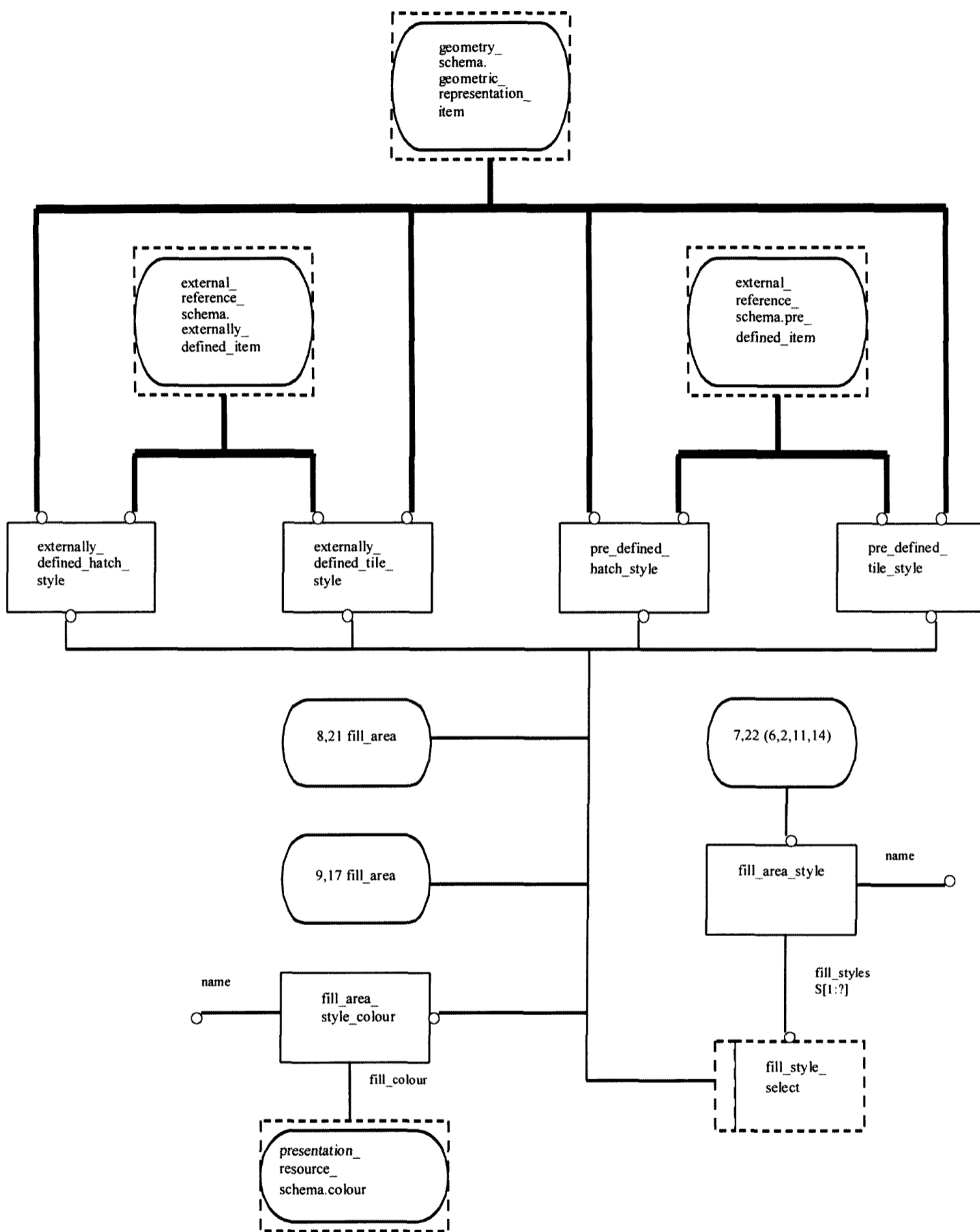
Рисунок E.23 — EXPRESS-G диаграмма presentation_appearance_schema 7 из 21
