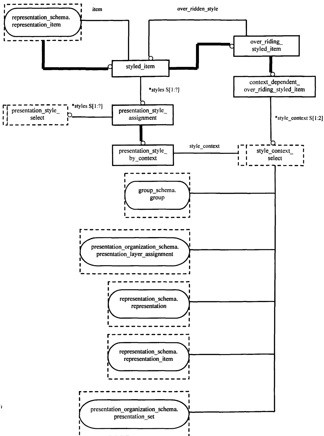
Рисунок E.17 — EXPRESS-G диаграмма presentation_appearance_schema 1 из 21
