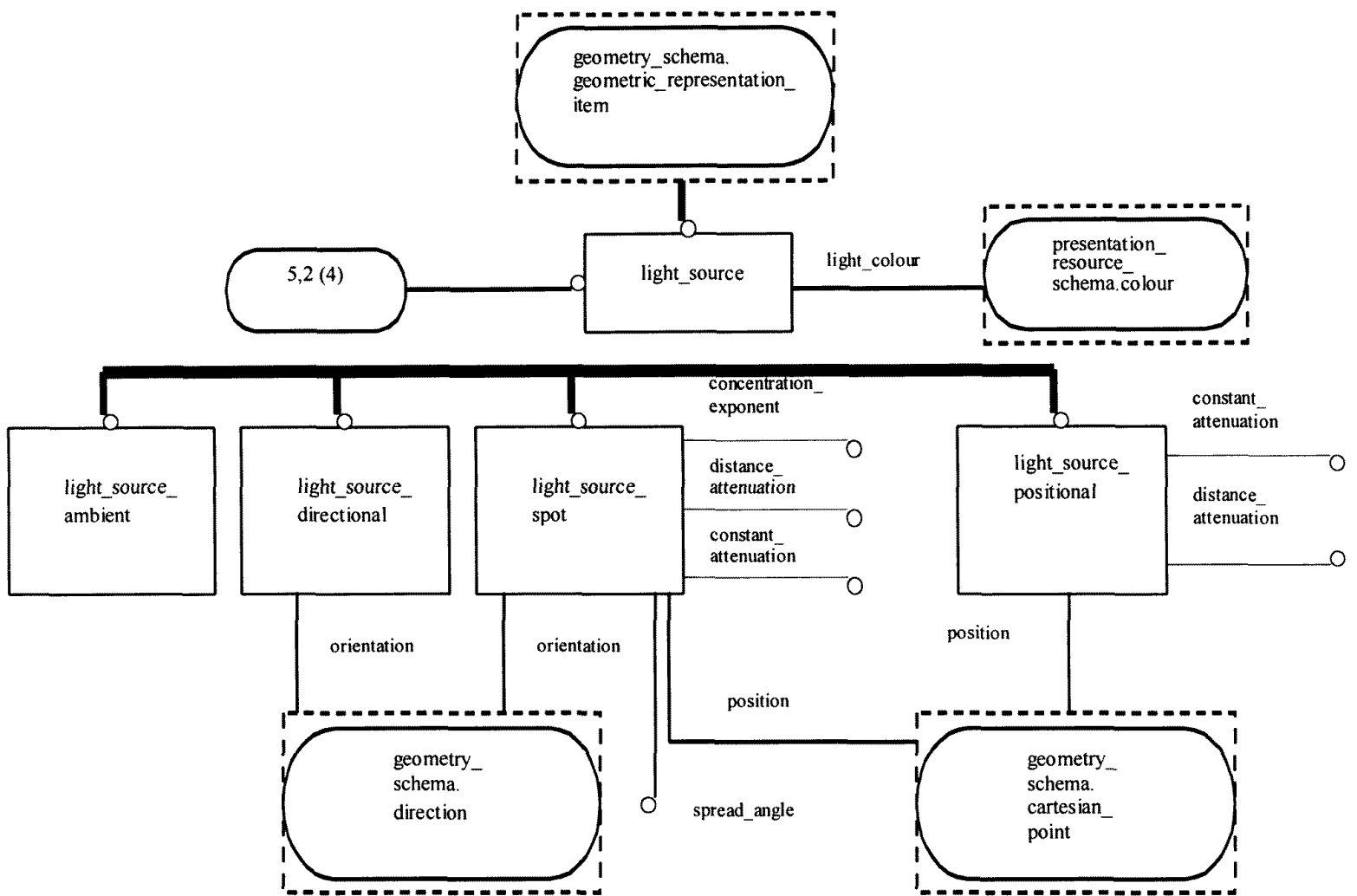
Рисунок Е.5 — EXPRESS-G диаграмма presentation_organization_schema 5 из 7
