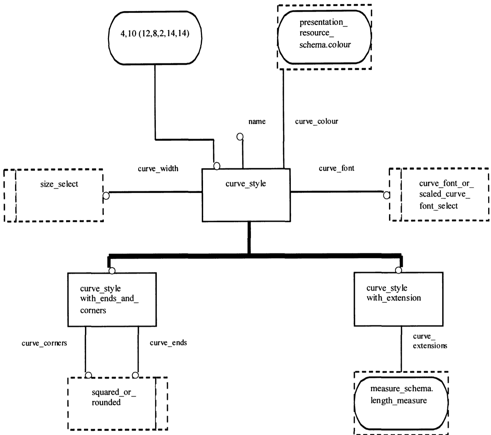
Рисунок E.20 — EXPRESS-G диаграмма presentation_appearance_schema 4 из 21
