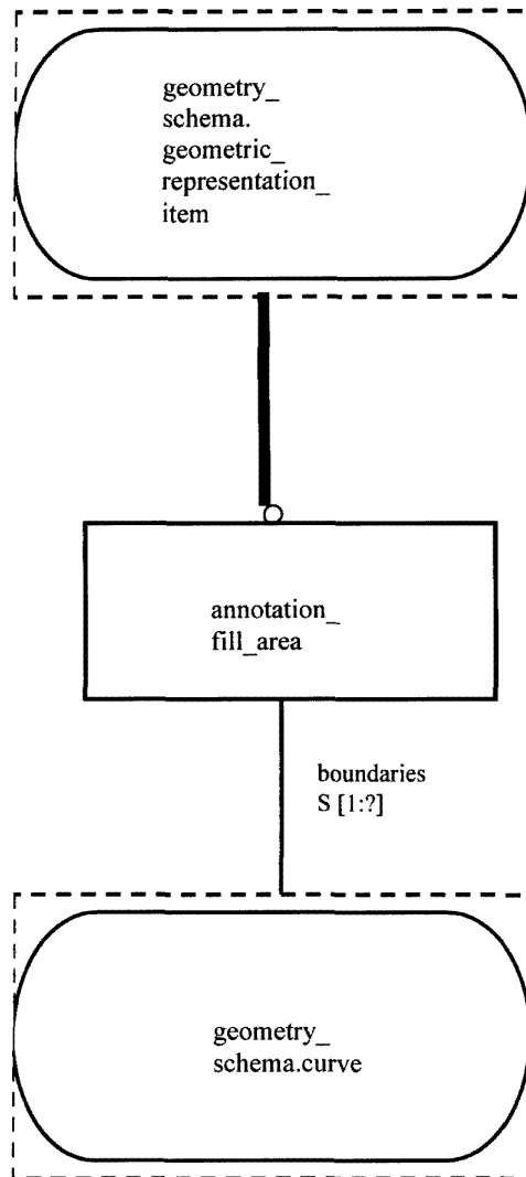
Рисунок Е.8 — EXPRESS-G диаграмма presentation_definition_schema 1 из 9
