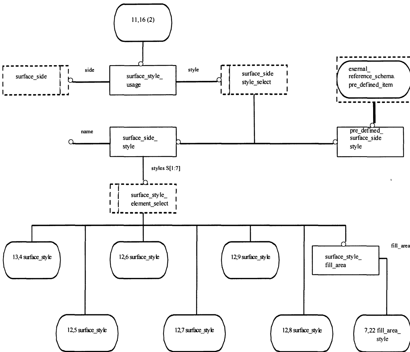
Рисунок E.27 — EXPRESS-G диаграмма presentation_appearance_schema 11 из 21
