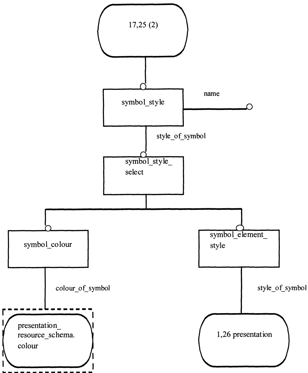
Рисунок Е.33 — EXPRESS-G диаграмма presentation_appearance_schema 17 из 21
