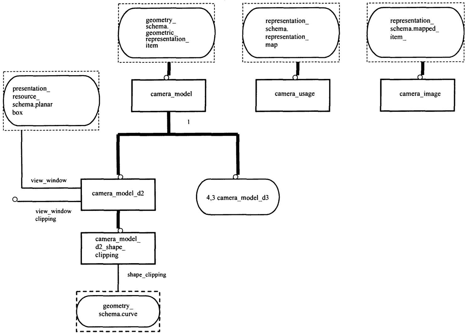
Рисунок Е.3 — EXPRESS-G диаграмма presentation_organization_schema 3 из 7
