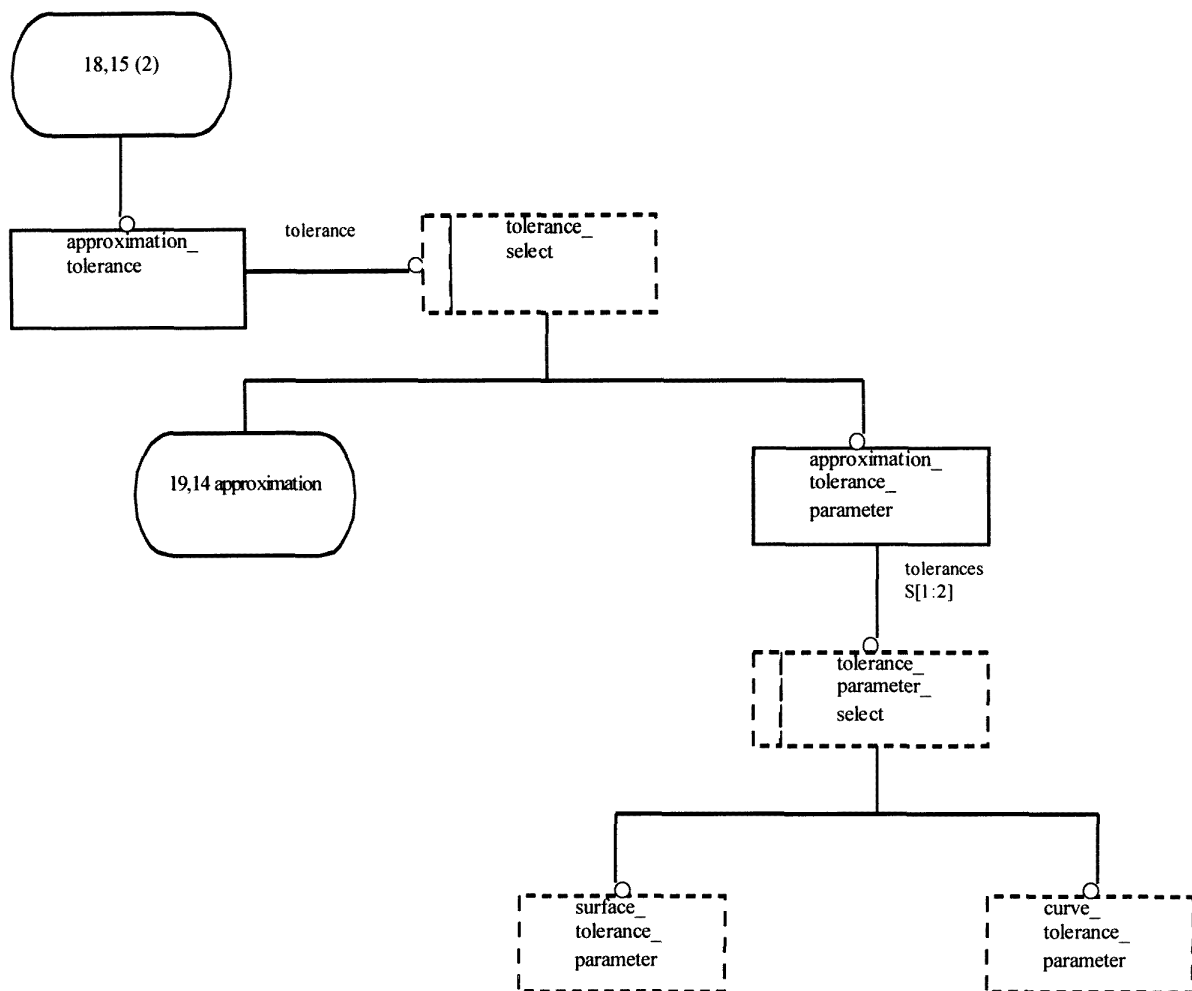
Рисунок Е.34 — EXPRESS-G диаграмма presentation_appearance_schema 18 из 21
