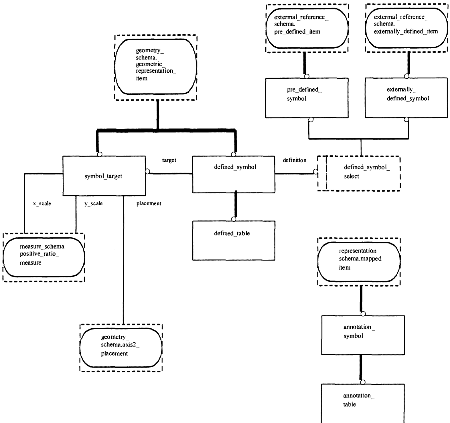
Рисунок Е.9 — EXPRESS-G диаграмма presentation_definition_schema 2 из 9
