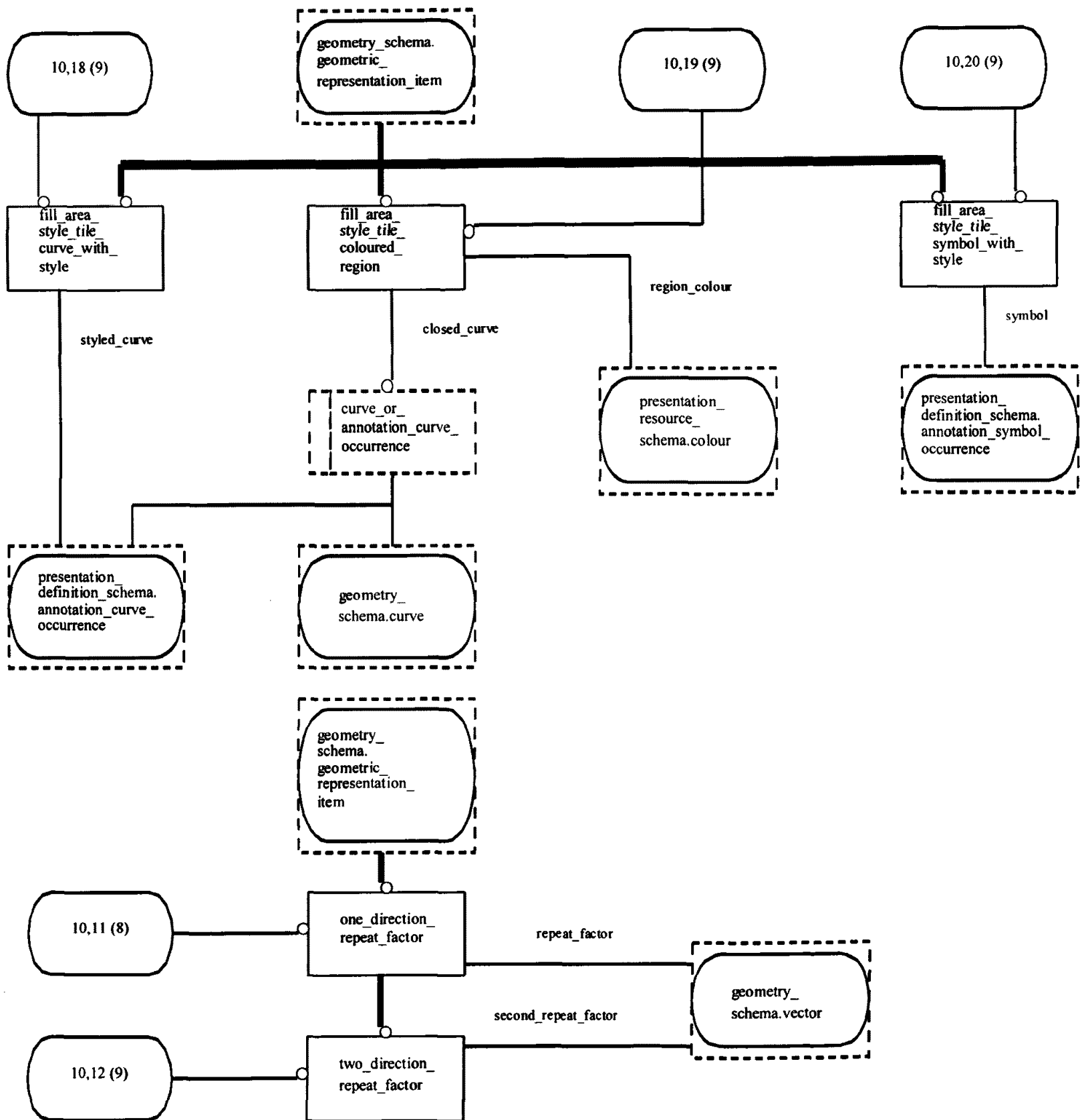
Рисунок E.26 — EXPRESS-G диаграмма presentation_appearance_schema 10 из 21
