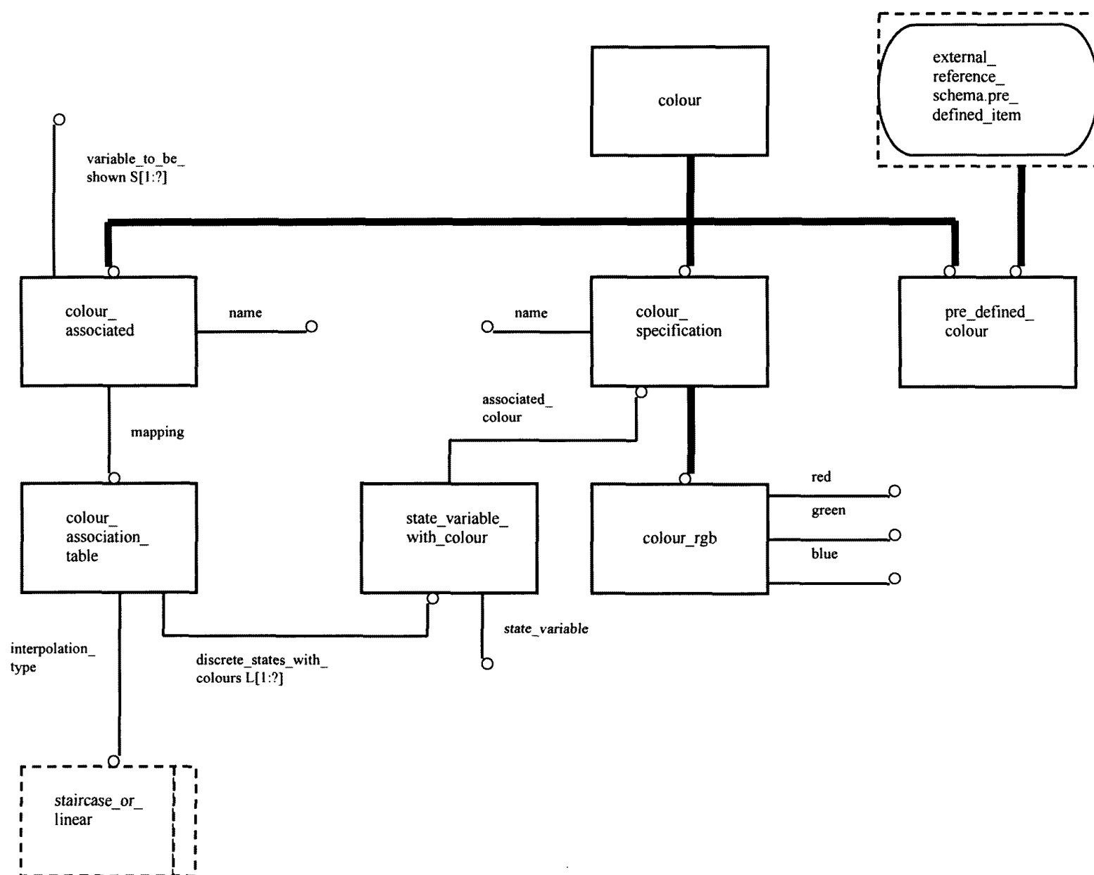
Рисунок Е.41 — EXPRESS-G диаграмма presentation_resource_schema 4 из 5
