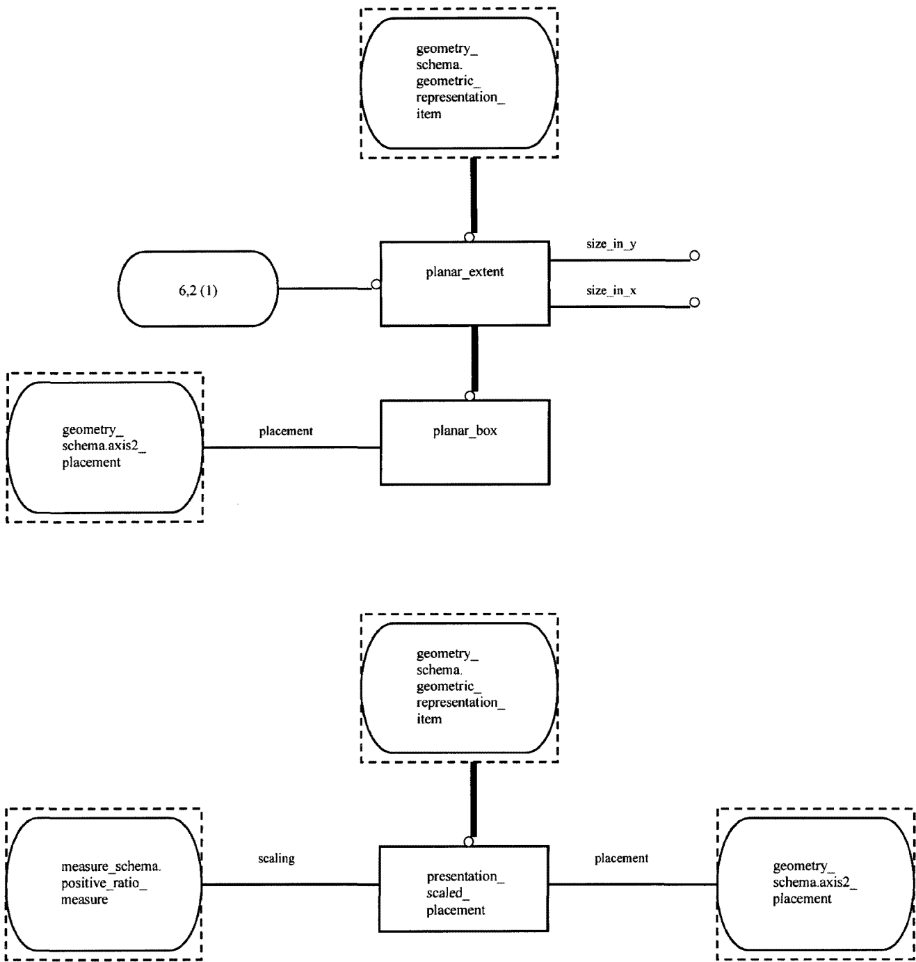
Рисунок Е.42 — EXPRESS-G диаграмма presentation_resource_schema 5 из 5
