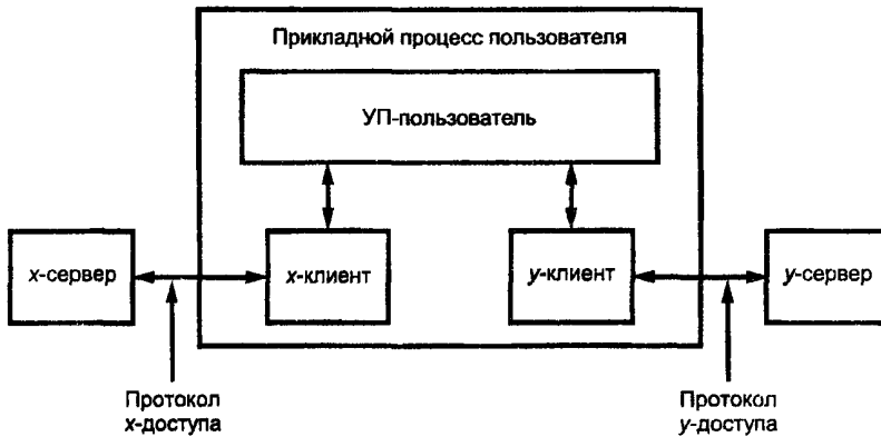
Рисунок D.5 — Несколько распределенных учрежденческих приложений
