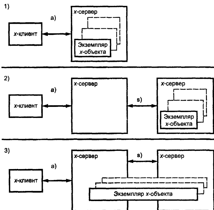
Рисунок J 1 — Сервер и экземпляры объектов
