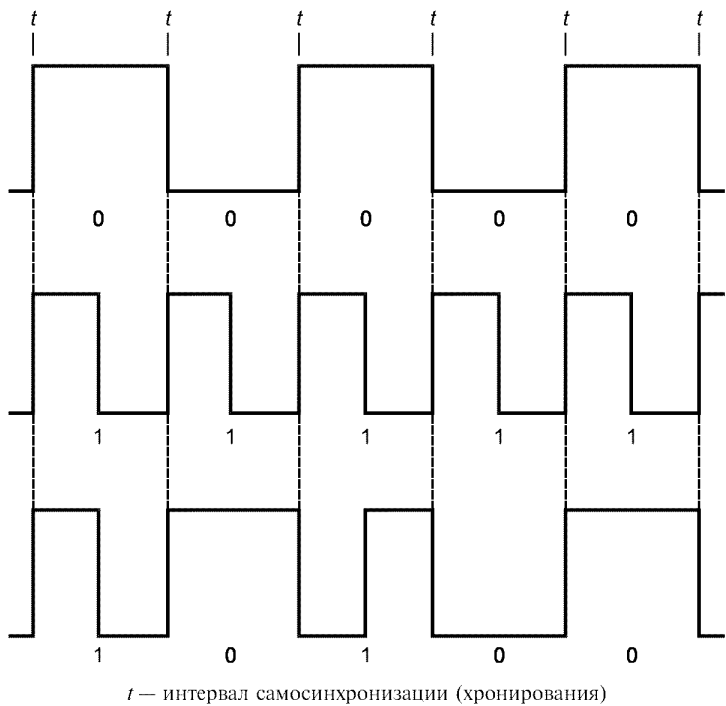
Рисунок 8 — Пример двухчастотного синфазного кодирования
