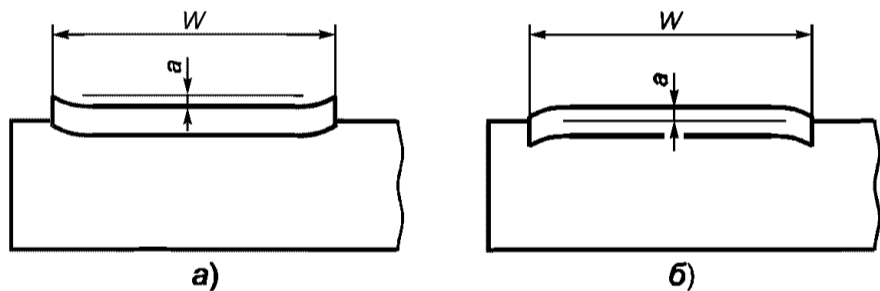
Рисунок 3 — Профиль поверхности
