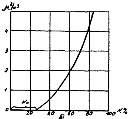
Типовая рабочая характеристика дымомера.
