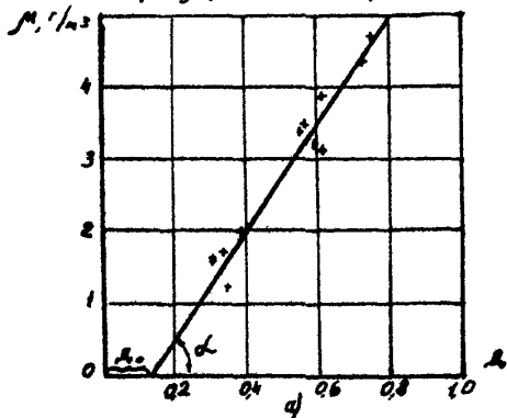
Типовая градуировочная характеристика дымомера
