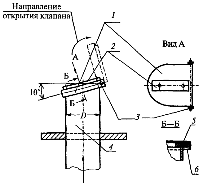
Рис. 3. Конструктивная схема взрыворазрядного устройства с откидным клапаном и вертикальным отводящим трубопроводом:
