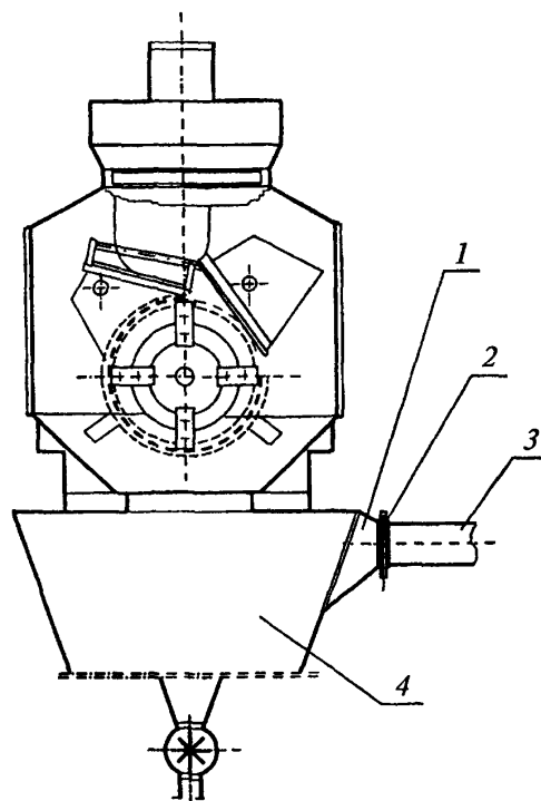
Рис. 17. Схема расположения взрывовзрядного устройства на поддобильном бункере:
