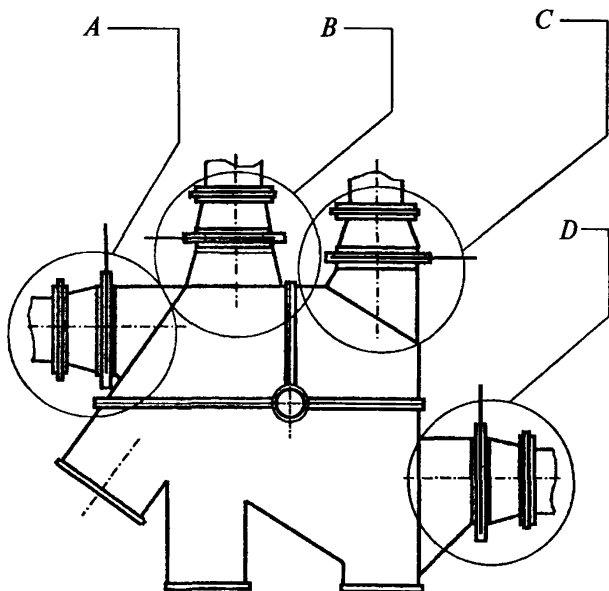
Рис. 10. Возможные варианты расположения взрыворазрядных устройств на головке нории с гравитационной разгрузкой: A, D — взрыворазрядные устройства с горизонтальными отводящими трубопроводами; B, C — взрыворазрядные устройства с вертикальными отводящими трубопроводами
