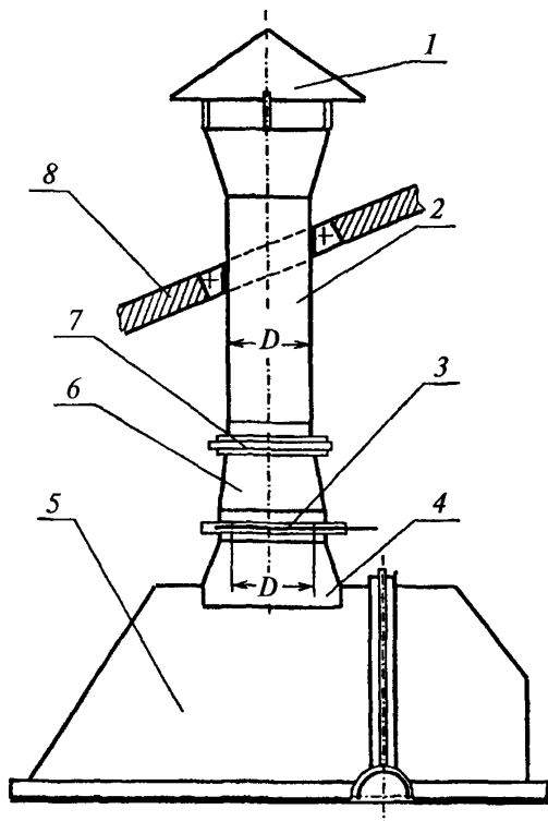
Рис. 9. Схема расположения на головке норрии взрыворазрядного устройства шиберного типа:
