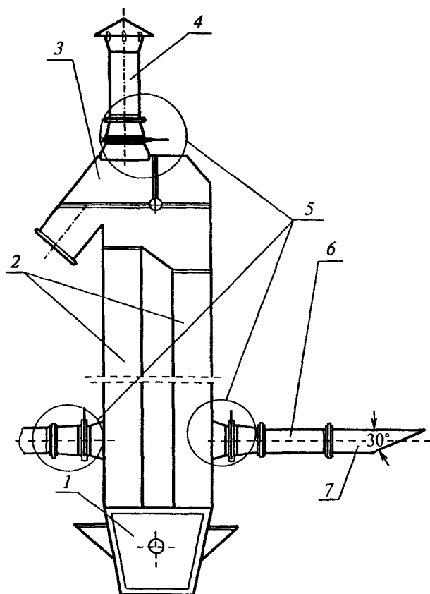
Рис. 8. Схема расположения на нории взрывозрядных устройств шиберного типа:
