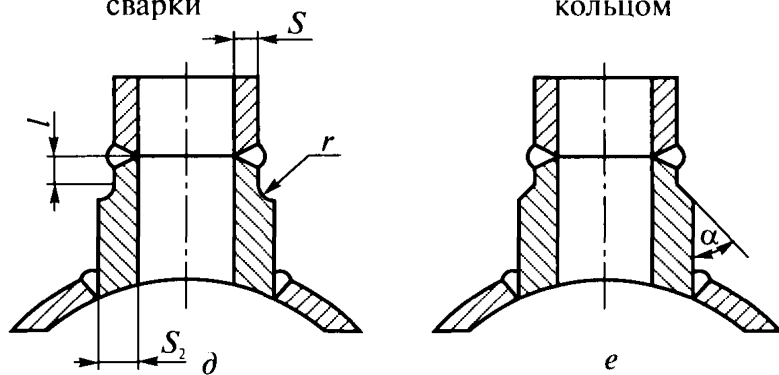
Рис. 14. Стыковка элементов разной толщины
