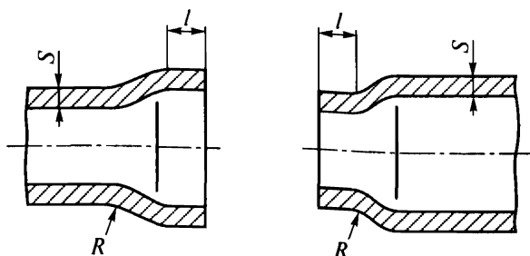
Рис. 5. Отбортованный и переходный элемент
