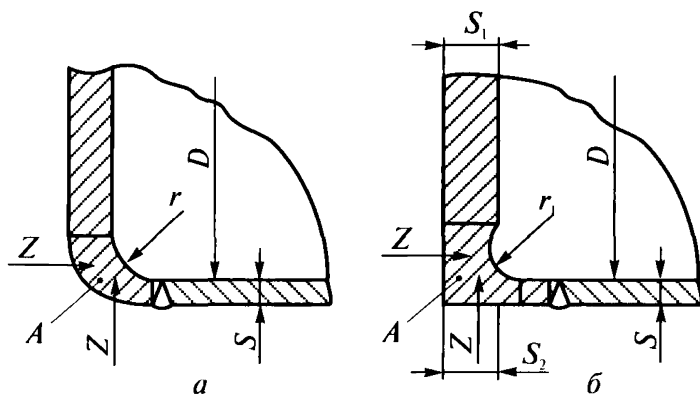
Рис. 4. Плоские днища
