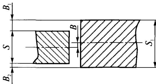
Рис. 15. Смещение кромок
