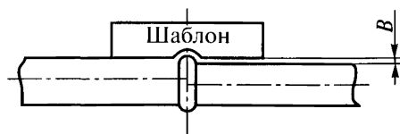
Рис. 10. Схема определения смещения кромок стыкуемых труб
