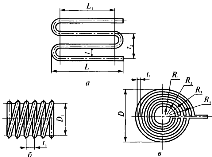
Рис. 12. Размеры гнутых змеевиков
