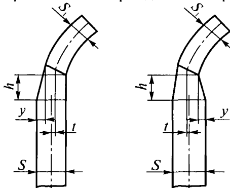
Рис. 2. Узел соединения днища с обечайкой
