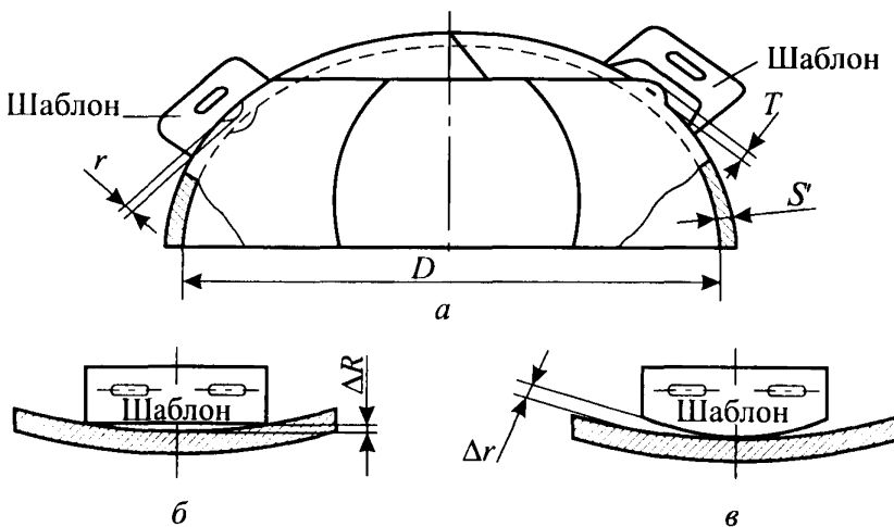
Рис. 7. Отклонение формы полусферического днища
