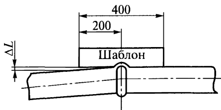
Рис. 11. Схема определения отклонения от прямолинейности оси трубы
