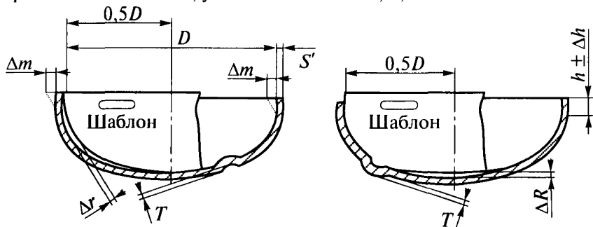
Рис. 6. Отклонение размеров и формы эллиптического днища
