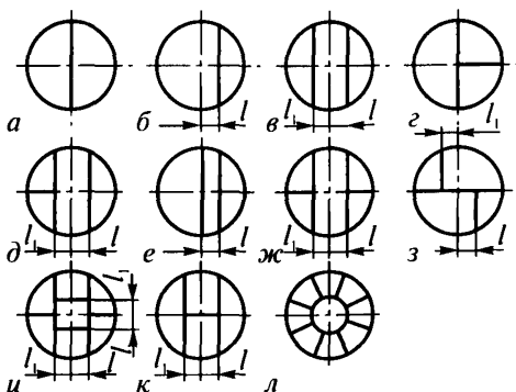
Рис. 1. Расположение сварных швов заготовок выпуклых днищ
