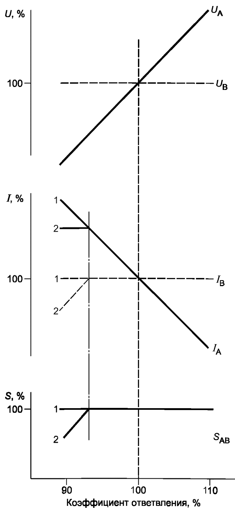
Рисунок 1 — Регулирование напряжения при постоянном магнитном потоке (режим a )
