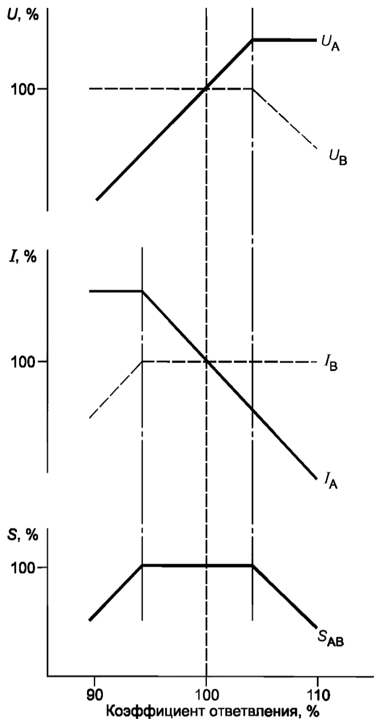
Рисунок 3 — Комбинированное регулирование напряжения (режим v )
