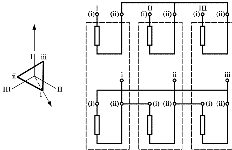
Рисунок Г.4 — Схема и группа соединения обмоток трехфазной группы однофазных трансформаторов (условное обозначение — Y/\Delta-5 )
