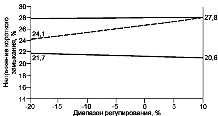
Рисунок В.1 — Диапазон изменения напряжения короткого замыкания
