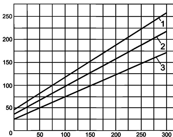
Рисунок С.1 — График зависимости силы торможения от усилия, приложенного к педали, выраженный «оптимальной прямой» и прямыми допусаемых предельных отклонений \pm 20\%
