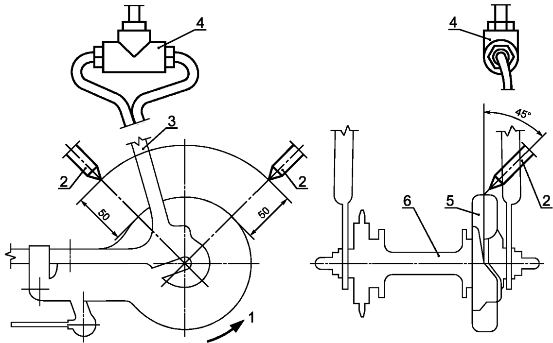
1 — направление вращения колеса; 2 — патрубок; 3 — рама; 4 — задний тройник; 5 — ленточный тормоз; 6 — задняя втулка Рисунок 9 — Патрубки для подачи воды для ленточного тормоза
