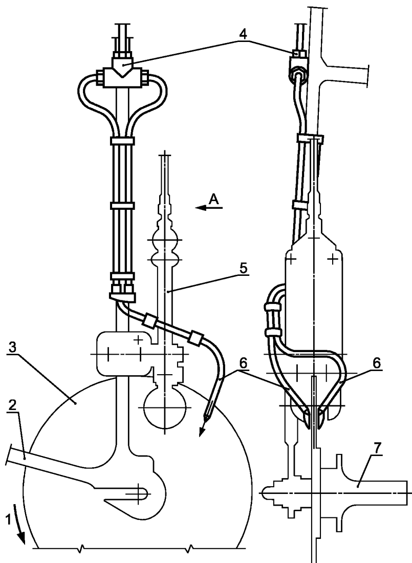
1 — направление вращения колеса; 2 — патрубок; 3 — рама; 4 — задний тройник; 5 — ленточный тормоз; 6 — задняя втулка Рисунок 9 — Патрубки для подачи воды для ленточного тормоза
