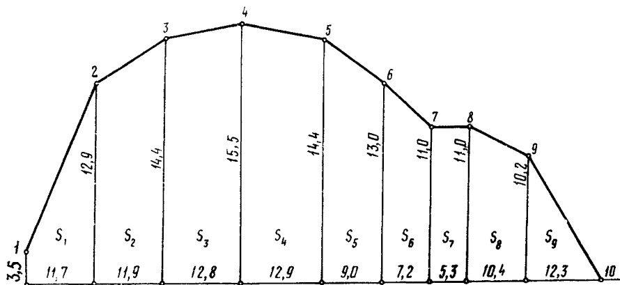
Рис. 8. Пример вычисления площади профиля аналитическим методом:
