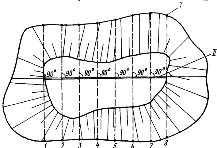
Рис. 5. Схема расположения параллельных линий при отсутствии пунктов съемочного обоснования: 1-8 - параллельные профильные линии; 1 - пикет на профильной линии; I - исходная базисная линия
