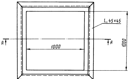
Рис. 1. Измерительная рамка
