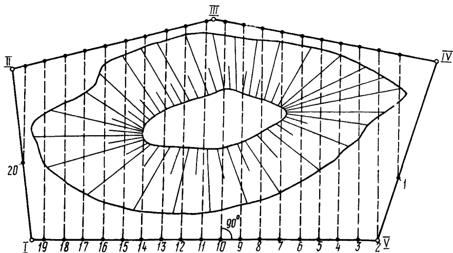
Рис. 4. Схема расположения профильных линий при неправильной форме штабеля: 1-20 - параллельные профильные линии; 1-V - основные пункты съемочного обоснования
