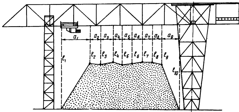
Рис. 7. Пример измерения высоты штабеля с крана-перегрузателя
