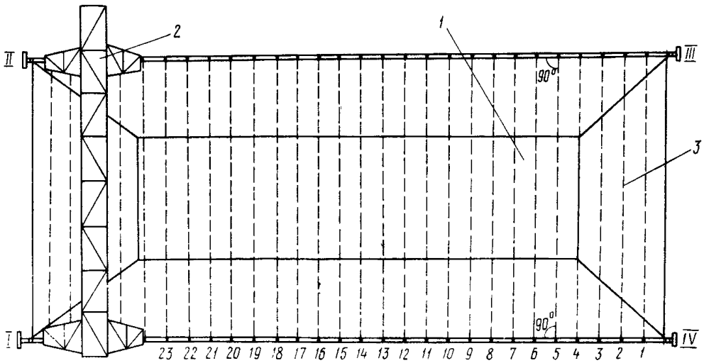
Рис. 3. Схема расположения профильных линий на штабеле топлива, обслуживаемом краном-перегрузателем: 1 - штабель; 2 - кран-перегрузатель; 3 - параллельные профильные линии; 1-1У - основные пункты съёмочного обоснования
