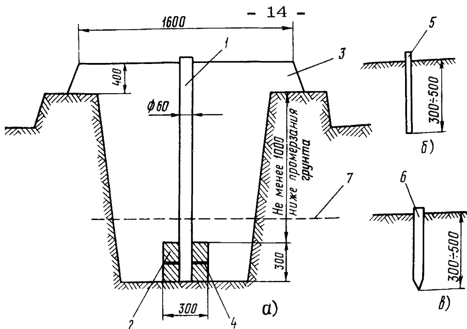
Рис. 2. Знаки съемочного обоснования:
