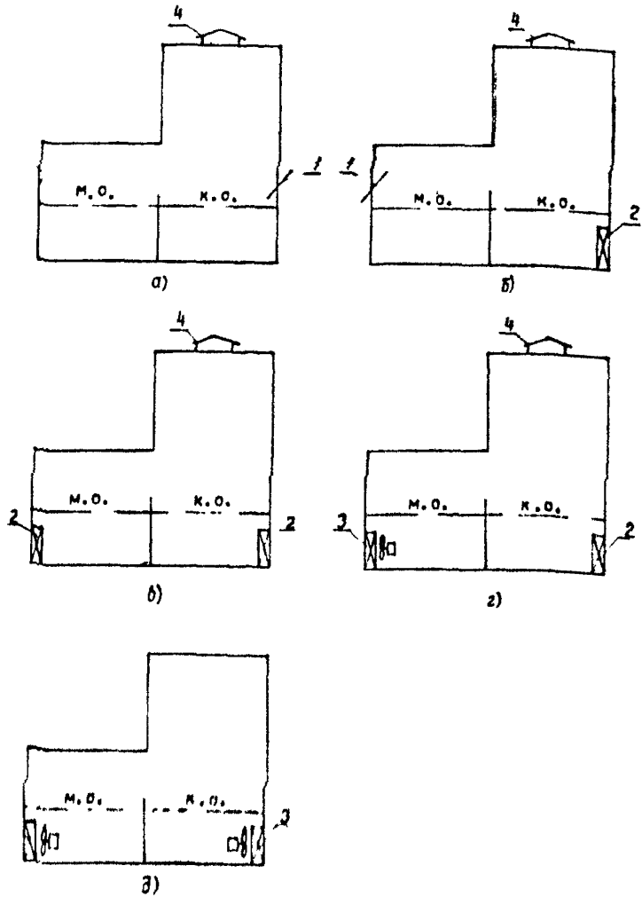
Рис. I. Схемы общеобменной вентиляции главных корпусов тепловых электростанций:
