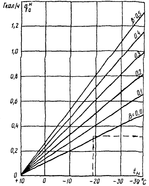
Рис.11. Зависимость нормы расхода тепла на отопление машинного отделения от t_H и \beta
