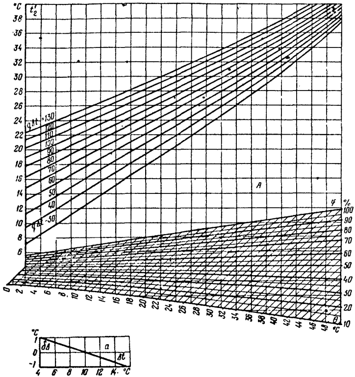
Рис.3. Нормативная характеристика башенной градирни площадью орошения 4000 м 2 с двухъярусным оросителем высотой 2,52 м (2-1,2+0,12) в расстоянии в свету между асбестоцементными щитами 19 мм
