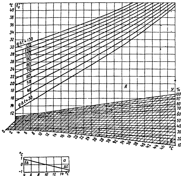
Рис.7. Нормативная характеристика бешенной грядки площадью орошения 1600 м 2 с двухъярусным оросителем высотой 2,45 м (2·1,2+0,05) в расстоянии между всбестопоментными штырями 40 мм, а также других различных грядок согласно табл.1
