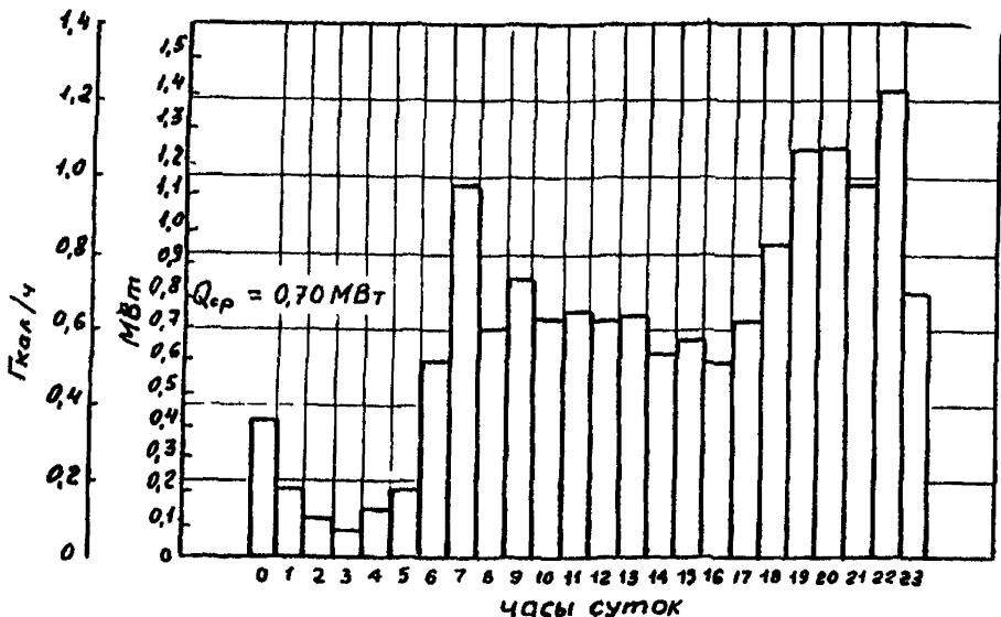
Рисунок Р3 - Изменение расхода тепла на горячее водоснабжение в течение суток
