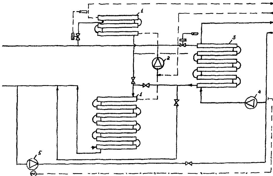
1 – подогреватель горячего водоснабжения № 12 ОСТ-34-588-68, I ступень – 7 секций II ступень – 3 секции 2 – циркуляционный насос К-90/20, 3 шт, 3 – подогреватель отопления № 14 ОСТ-34-588-68, 6 секций, 4 – отопительные насосы К-90/55А, 5 – подпиточный насос ВК 2х2В, 2 шт Рисунок Р 1 – Принципиальная тепловая схема ЦТП
