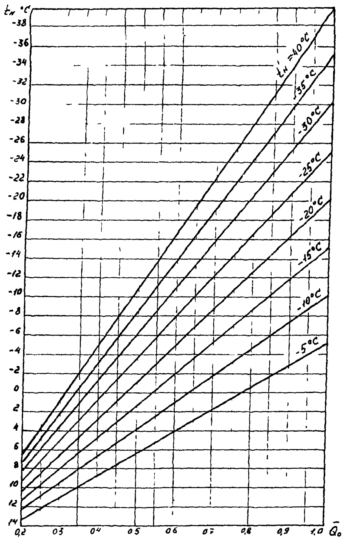
Рисунок Л4 Зависимость температур наружного воздуха t_n от расчетной относительной нагрузки отопления \bar{Q} , при разных значениях расчетной для отопления температуры наружного воздуха t_n
