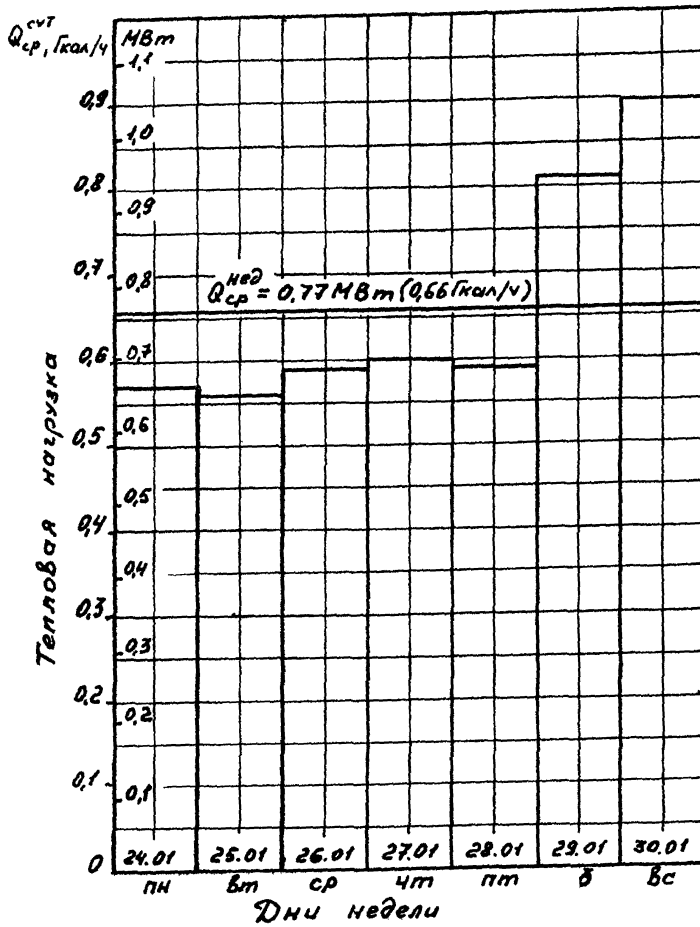
Рисунок Р4 - ЦТП Среднесуточные нагрузки горячего водоснабжения
