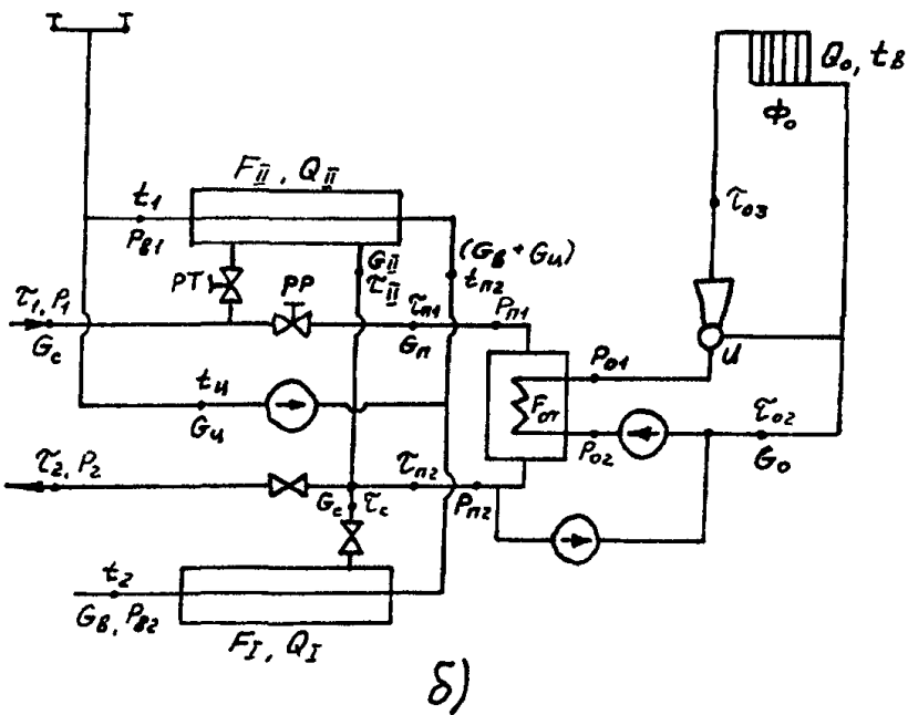
Рисунок 1 Схемы тепловых пунктов
