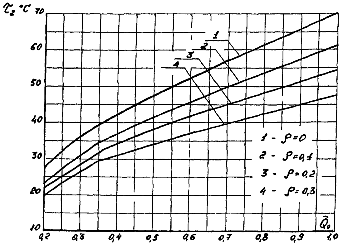
Рисунок 12 лист 4 Температурный график повышенный рассчитанный на \mu = 0,3
