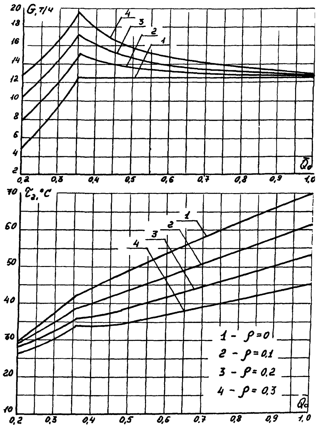
Рисунок Л.3 - Требуемые расходы и температуры обратной сетевой воды при средней нагрузке горячего водоснабжения. Схема присоединения системы отопления - зависимая. Схема присоединения нагрузки горячего водоснабжения - смешанная. Температурный график - отопительный
