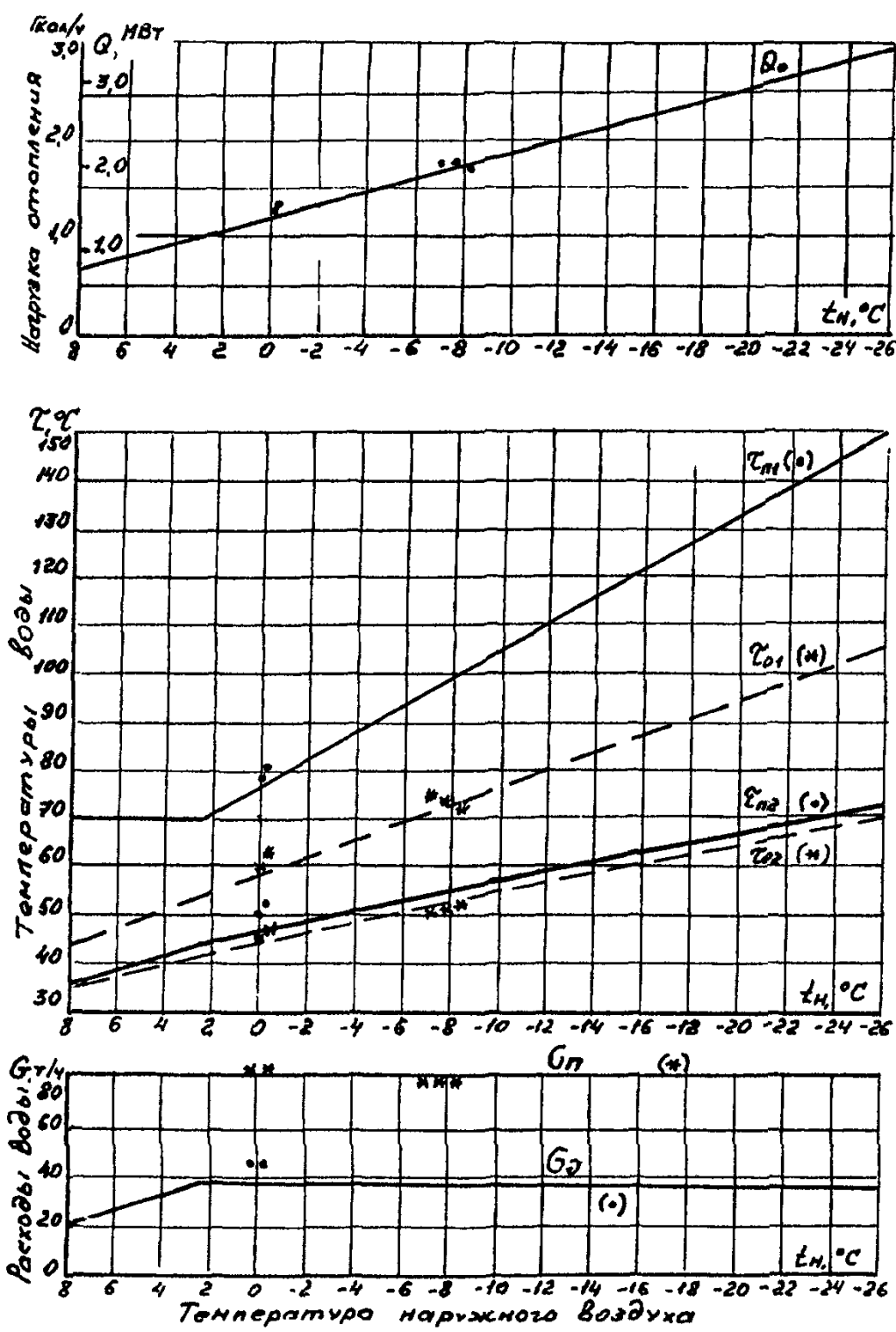
Рисунок Р 2 – Режимы работы системы отопления при проектной нагрузке Q'_0=3,41 МВт
