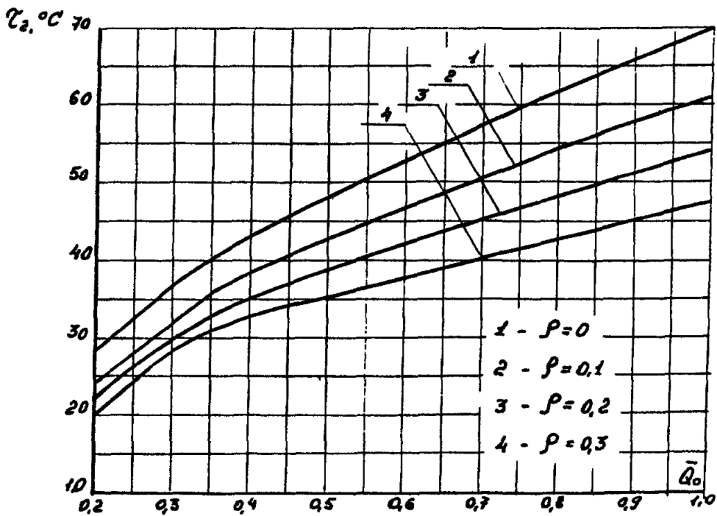
Рисунок Л.2, лист 2 Температурный график повышенный, рассчитанный на \rho = 0.2
