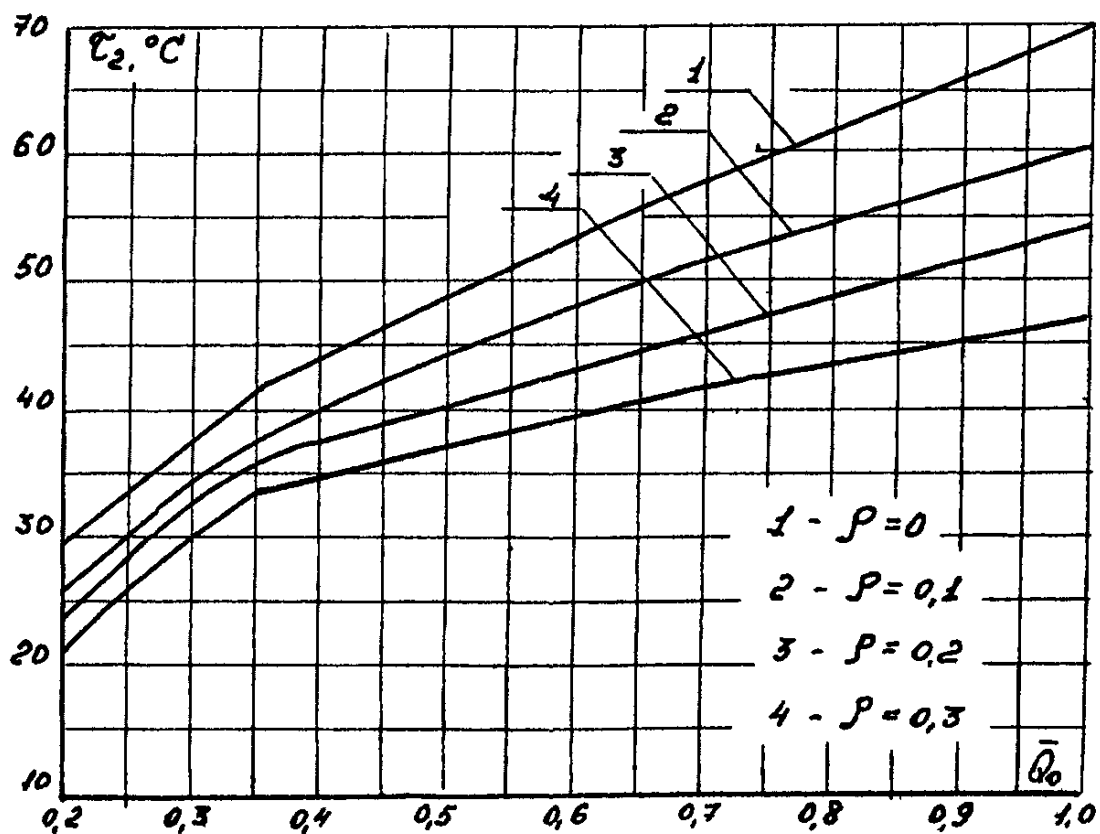
Рисунок Л 2, лист 1 Требуемые расходы и температуры обратной сетевой воды при средней нагрузке горячего водоснабжения. Схема присоединения системы отопления — зависимая. Схема присоединения нагрузки горячего водоснабжения — последовательная. Температурный график — отопительный.
