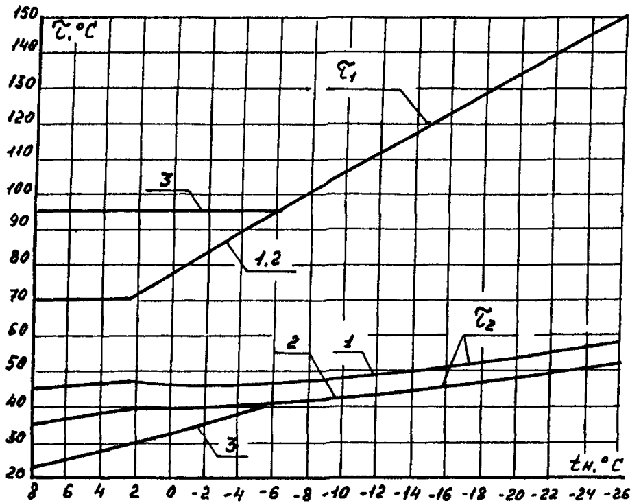
Рисунок Р7 - Режимы работы ЦТН при фактических гелловых нагрузках и проведении энергосберегающих мероприятия
