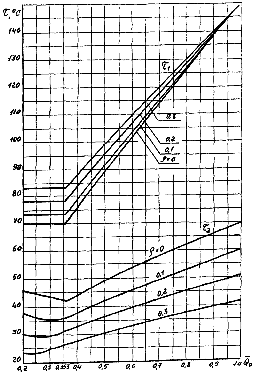
Рисунок Л.1 Отопительный и повышенные температурные графики
