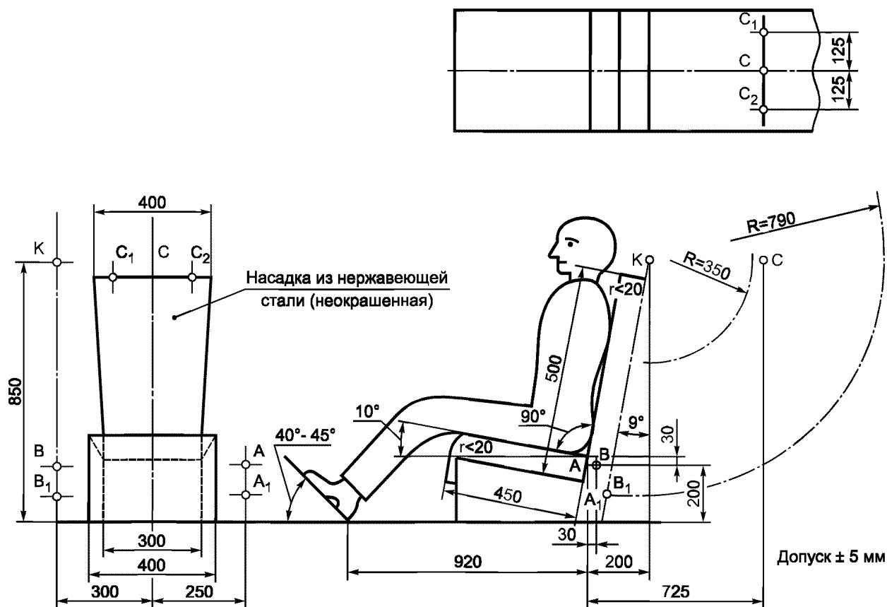
Рисунок 6.1 — Тележка, сиденье, приспособление для крепления ремня
