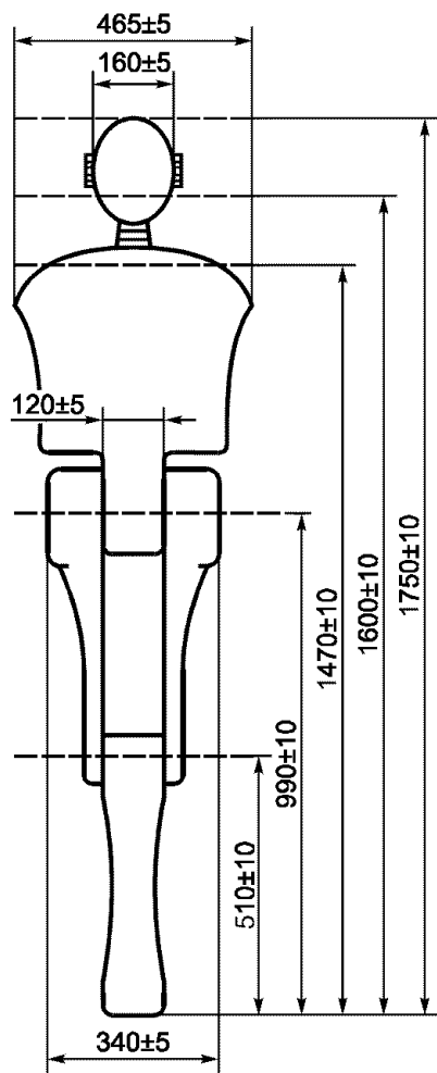
Рисунок 7.5 — Основные размеры
