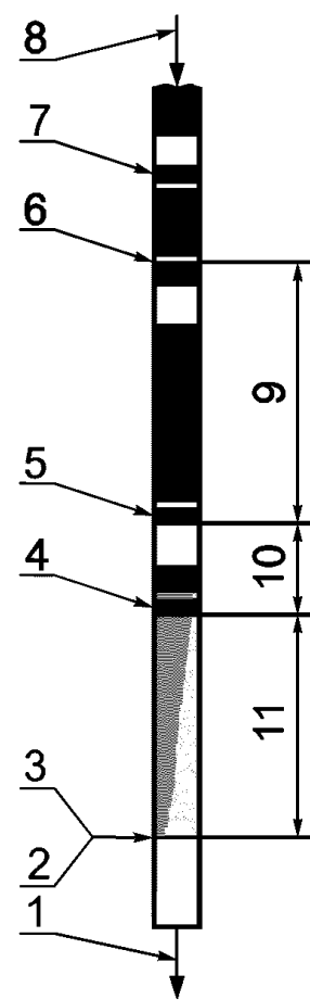
1 — нижняя часть; 2 — фронт элюирования; 3 — чистая жидкость; 4 — первая интенсивная желтая флуоресценция; 5 — первая интенсивная голубая флуоресценция; 6 — красно-коричневое кольцо; 7 — дополнительное красное кольцо; 8 — верхняя часть; 9 — зона ароматики; 10 — зона олефинов; 11 — зона насыщенных углеводородов
