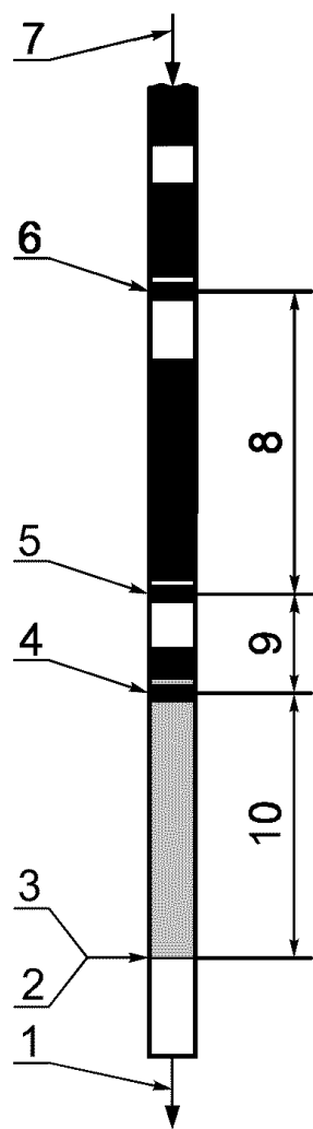
1 — нижняя часть; 2 — фронт элюирования; 3 — чистая жидкость; 4 — первая интенсивная желтая флуоресценция; 5 — первая интенсивная голубая флуоресценция; 6 — красное кольцо; 7 — верхняя часть; 8 — зона ароматических углеводородов; 9 — зона олефинов; 10 — зона насыщенных углеводородов
