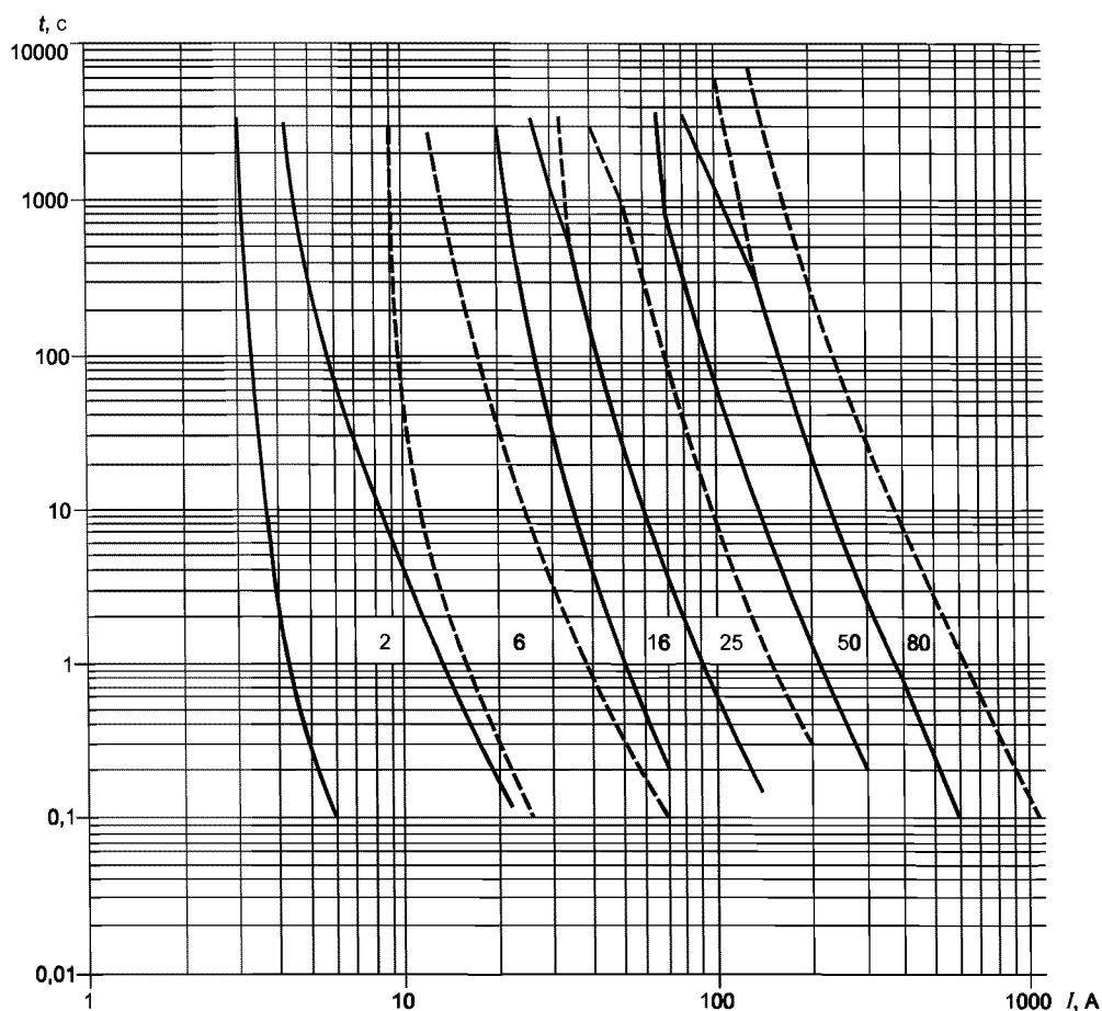
Рисунок А.1 — Времена-токовые зоны для плавкого предохранителя
