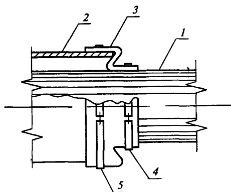
Рисунок 4 — Эластичное уплотнение на конце футляра
