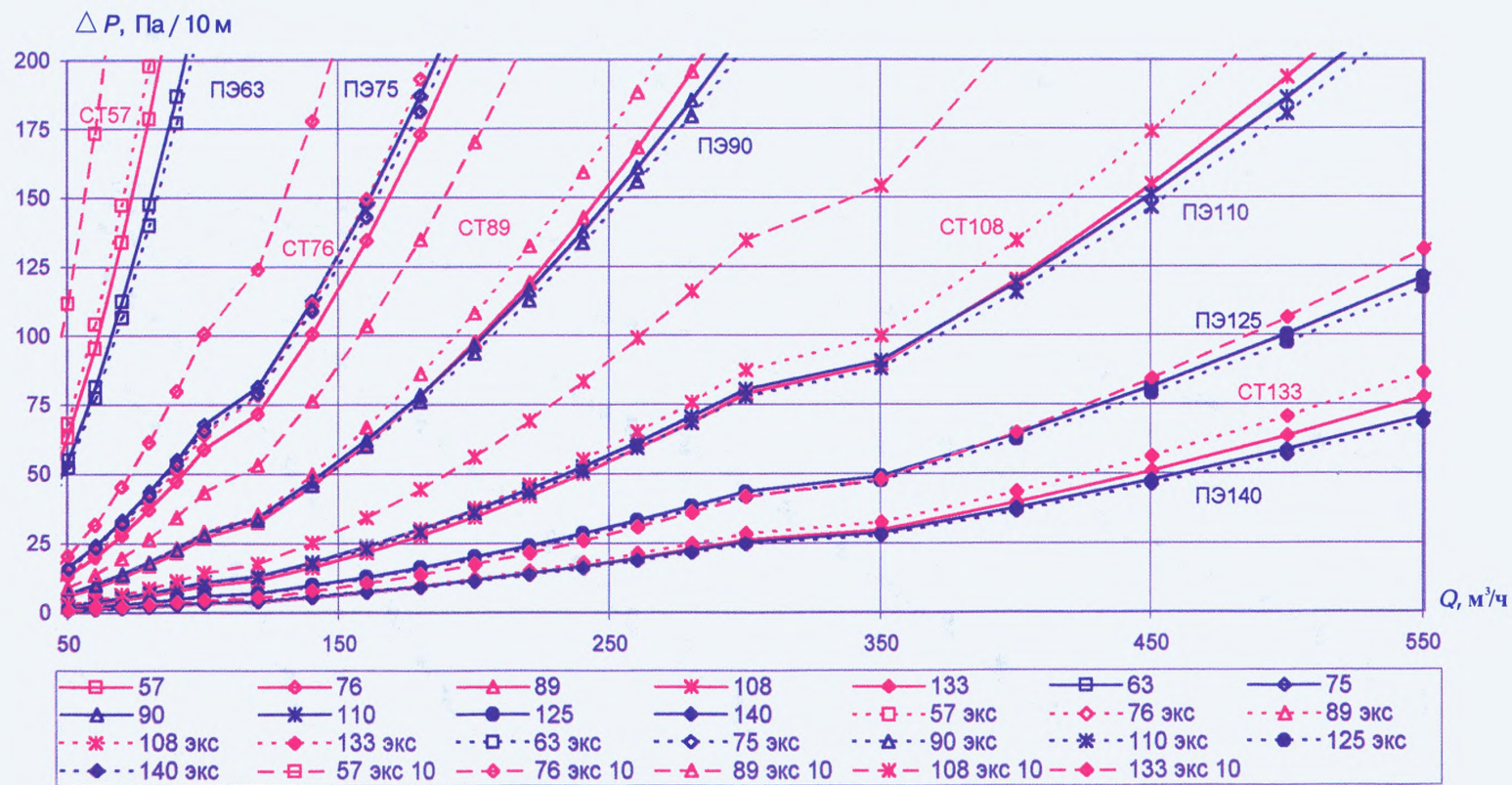
Удельные потери давления для стальных и полиэтиленовых труб (новых и бывших в эксплуатации) низкого давления (Q\ 50 - 500\ \text{м}^3/\text{ч}, \rho = 0,73\ \text{кг}/\text{м}^3, \nu = 1,4 \times 10^{-6}\ \text{м}^2/\text{с})
