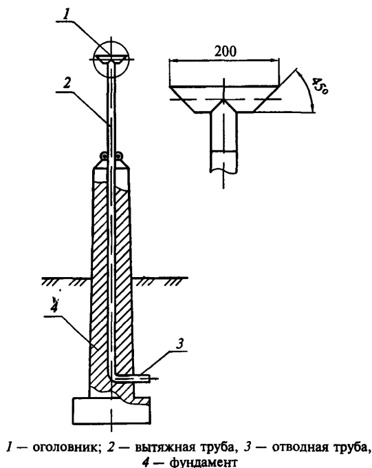
Рисунок 2 — Вытяжная свеча
