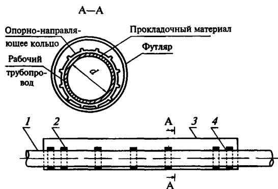
Рисунок 3 — Прокладка газопровода в футляре
