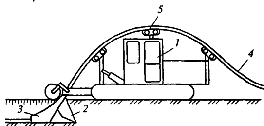
1 — гусеничный тягач, 2 — режущий нож, 3 — шнек, 4 — трубная плеть, 5 — роликоопора
