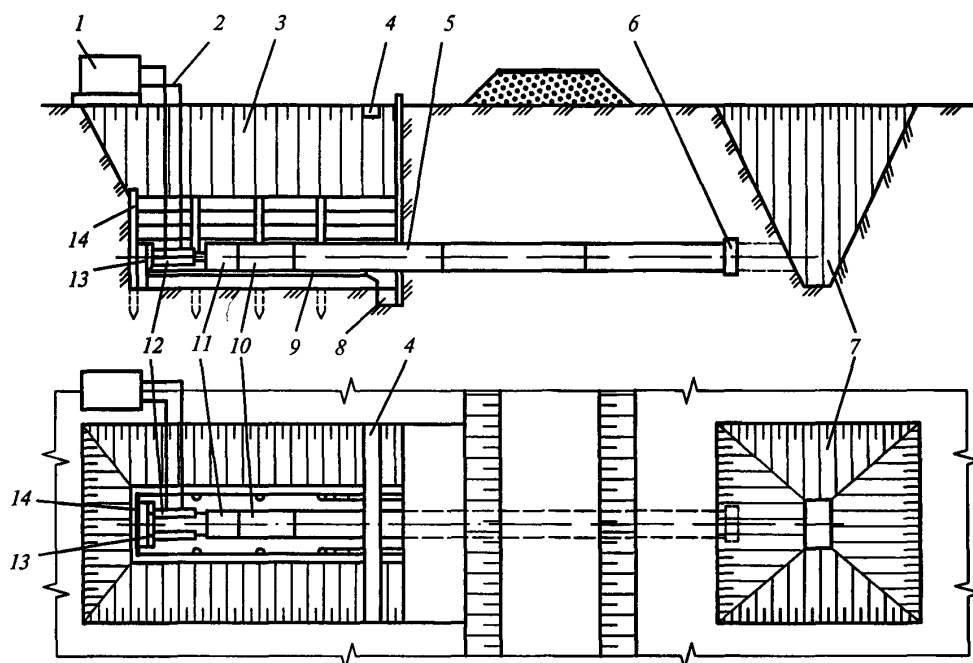
1 — насосная станция, 2 — газопровод, 3 — рабочий котлован, 4 — водоотводной лоток, 5 — защитный футляр, 6 — лобовая обделка (нож), 7 — приемный котлован, 8 — приемок для сварки защитного футляра, 9 — направляющая рама, 10 — нажимной патрубок, 11 — нажимная заглушка, 12 — гидродомкраты, 13 — башмак, 14 — упорная стенка
