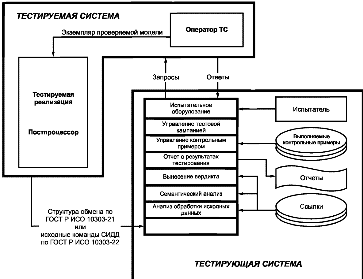
Рисунок 2 — Компоненты тестирования постпроцессора
