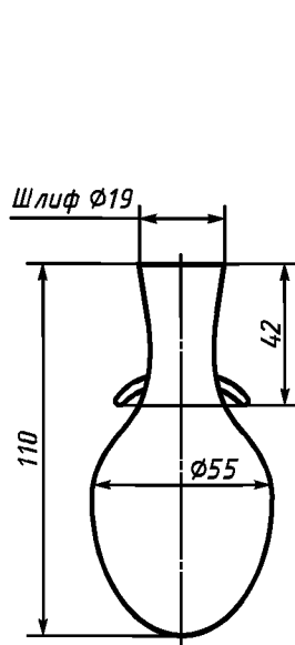
Рисунок В.4 — Реакционная колба
