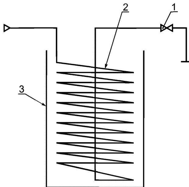
Рисунок 1 — Устройство для охлаждения сжиженного газа
