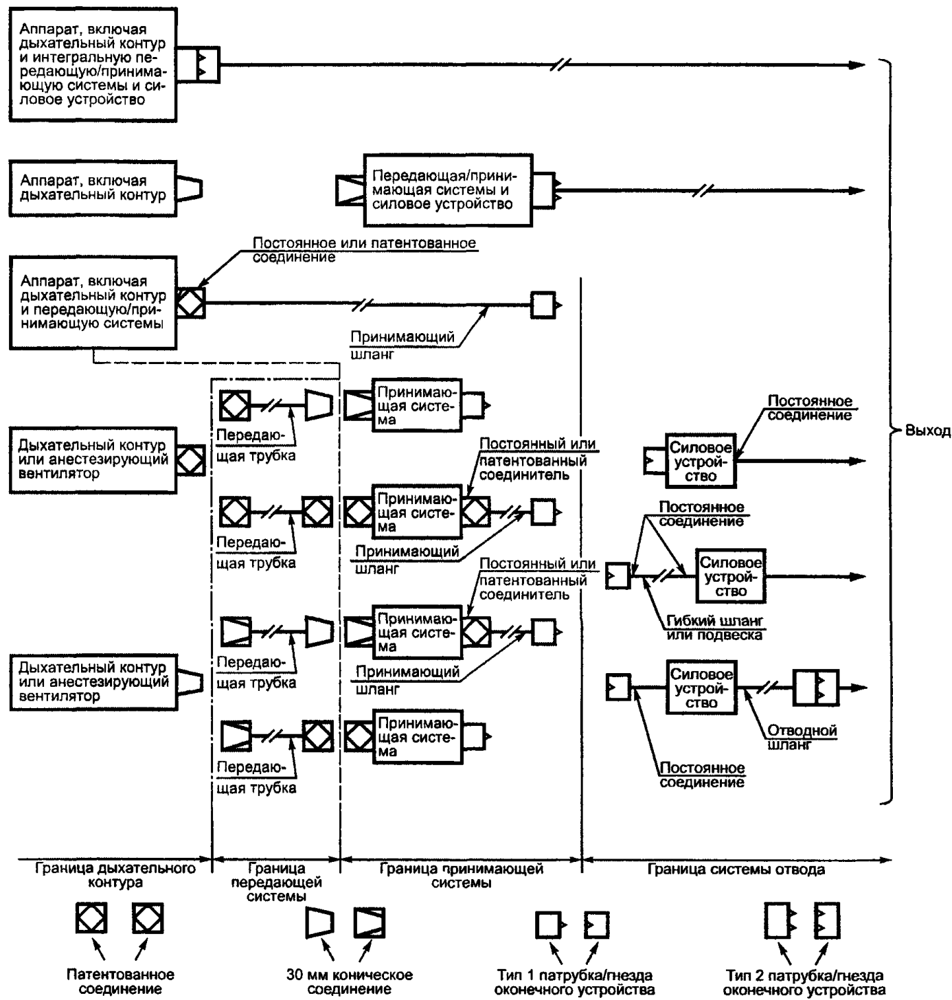
Рисунок 1 — Схема типичных соединений СВГС
