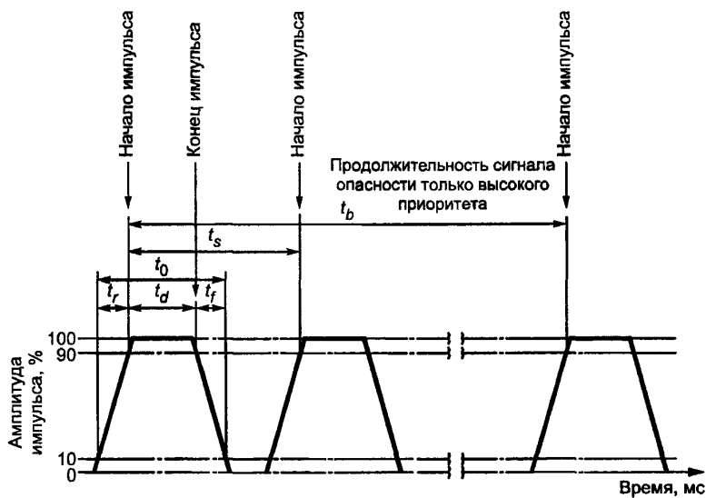
Рисунок 1 — Временные характеристики звуковых сигналов
