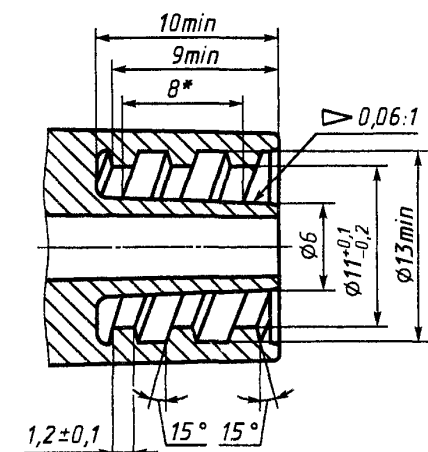
Рисунок 1 — Основные размеры соединителей на входе и выходе полости по крови
