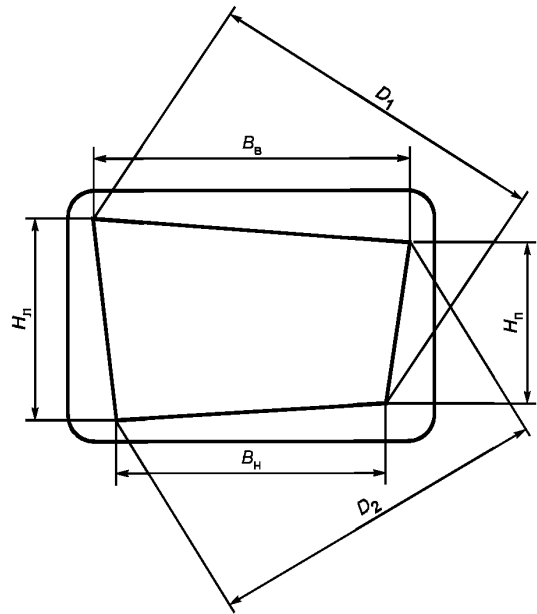
Рисунок 6 — Определение отклонения рабочего поля от прямоугольной формы
