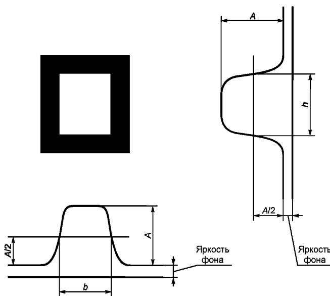
Рисунок 4 — Определение ширины и высоты знака по профилю яркости
