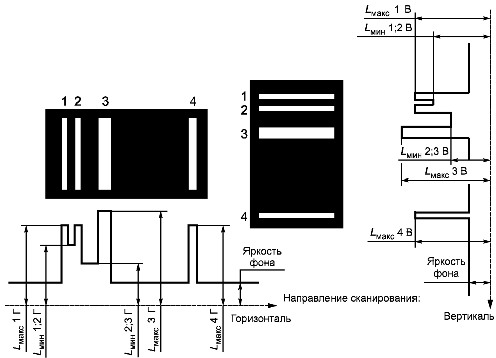
Рисунок 2 — Расположение штрихов и профили яркости тест-изображения
