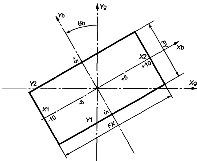
Угол поворота КОЛЛИМАТОРА ПУЧКА \theta_b = 30^\circ
