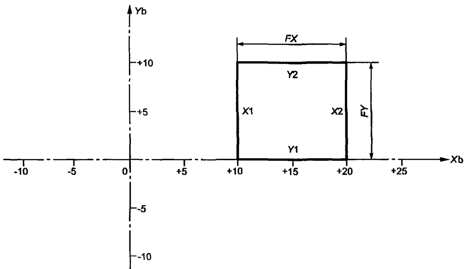
Угол поворота КОЛЛИМАТОРА ПУЧКА \theta_b = 0^\circ
