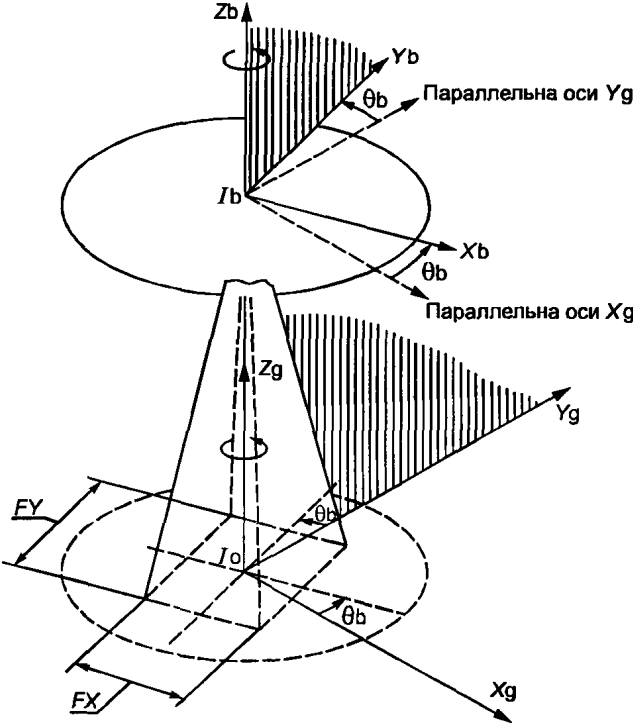
Рисунок 5 — Поворот на угол \theta_b = 15^\circ системы координат КОЛЛИМАТОРА ПУЧКА или ОГРАНИЧИТЕЛЯ ПУЧКА ИЗЛУЧЕНИЯ ( X_b, Y_b, Z_b ) в системе координат ШТАТИВА ( X_g, Y_g, Z_g ) и результирующее положение ПОЛЯ ОБЛУЧЕНИЯ (или ОГРАНИЧЕНИЯ ПОЛЯ ИЗЛУЧЕНИЯ) с размерами F_X и F_Y (см. 2.4)
