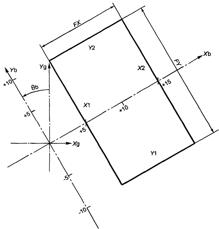
Угол поворота КОЛЛИМАТОРА ПУЧКА \theta_b = 30^\circ FX = 10 X1 = 5 X2 = 15 FY = 20
