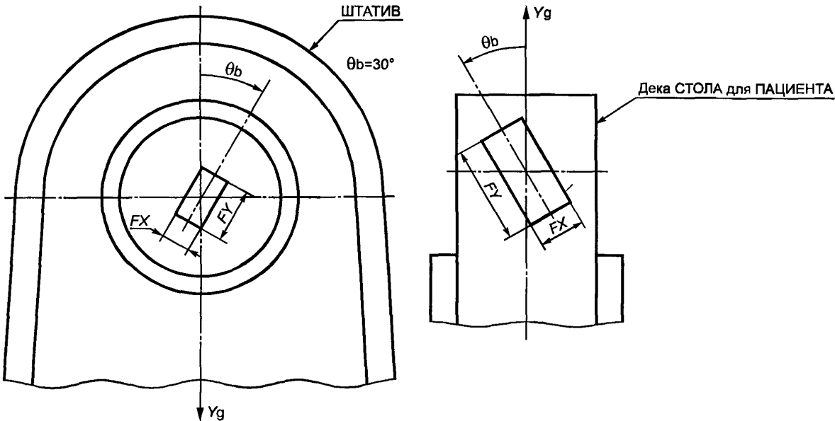
Рисунок 15а — Повернутое ( \theta_b = 30^\circ ) симметричное прямоугольное ПОЛЕ ОБЛУЧЕНИЯ ( F_X \times F_Y на стандартном расстоянии от ИСТОЧНИКА ИЗЛУЧЕНИЯ); вид из ИЗОЦЕНТРА в направлении ИСТОЧНИКА ИЗЛУЧЕНИЯ (см. 6.2)
