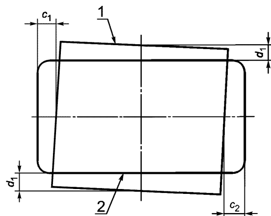
1 — ПОЛЕ РЕНТГЕНОВСКОГО ИЗЛУЧЕНИЯ; 2 — ПОВЕРХНОСТЬ ПРИЕМНИКА ИЗОБРАЖЕНИЯ
