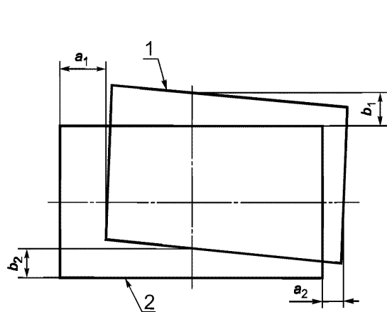
1 — визуально определенное поле; 2 — ПОЛЕ РЕНТГЕНОВСКОГО ИЗЛУЧЕНИЯ
