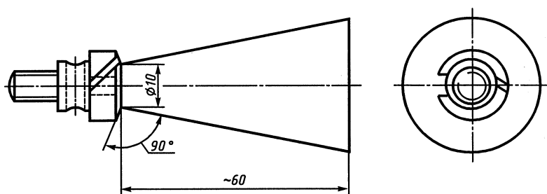
Рисунок 1 — Коническая оправка
