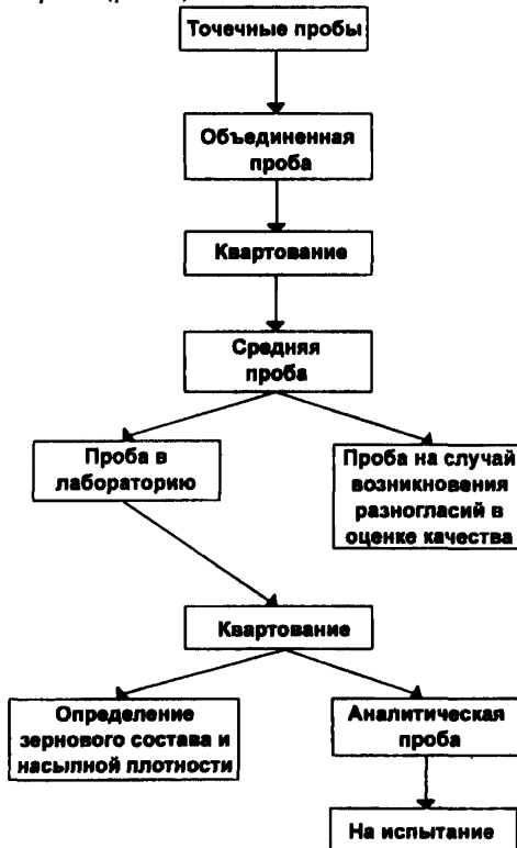
Рис. 1. Схема отбора и подготовки проб
