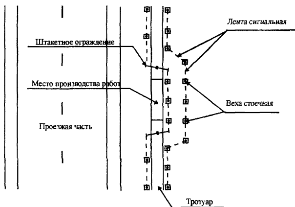
Рис. 12. Обозначение временного пешеходного пути с помощью вех и сигнального шнура
