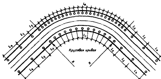
Рис. 10. Установка сигнальных столбиков в пределах кривых в плане
