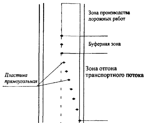
Рис. 11. Установка направляющих устройств в виде пластин на участке производства дорожных работ
