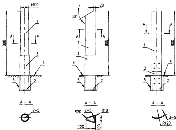
Рис. 4. Форма и размеры гибких составных ударобезопасных сигнальных столбиков из композиционных материалов 1 - верхняя часть корпуса столбика; 2 - нижняя часть корпуса столбика; 3 - гибкий эластичный узел; 4 - поверхность земли; 5 - опорная часть с удерживающим устройством
