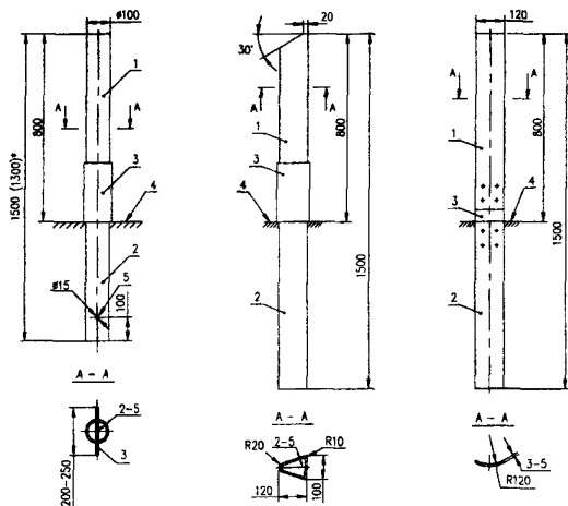
Рис. 3. Форма и размеры жестких сплошных ударобезопасных сигнальных столбиков из композиционных материалов 1 - верхняя часть корпуса столбика; 2 - нижняя часть корпуса столбика; 3 - гибкий эластичный узел; 4 - поверхность земли; 5 - анкерное устройство
