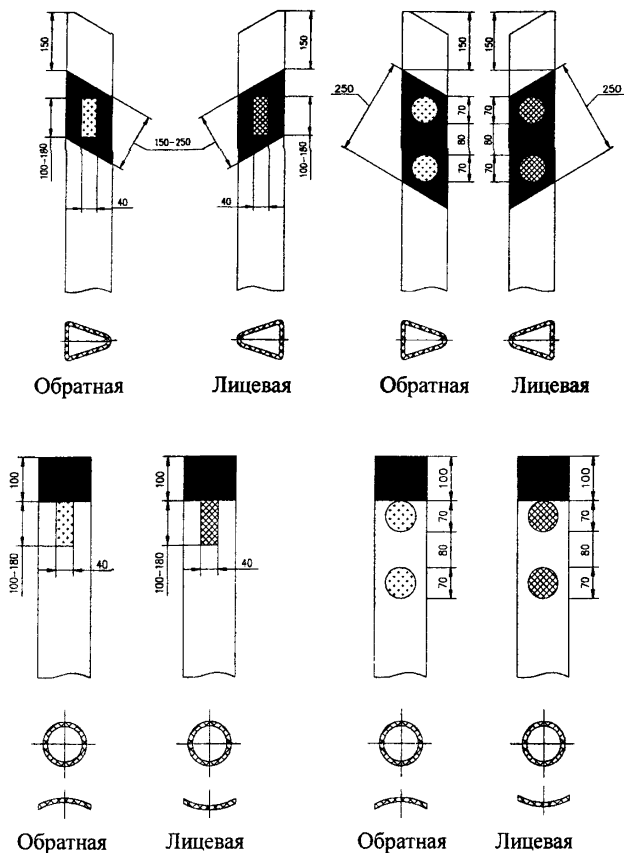
Рис. 5. Вертикальная разметка ударобезопасных сигнальных столбиков из композиционных материалов (лицевые и обратные стороны):
