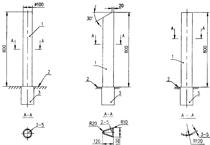
Рис. 2. Форма и размеры составных ударобезопасных сигнальных столбиков из композиционных материалов: 1 – корпус столбика; 2 – поверхность земли; 3 – опорная часть с удерживающим устройством
