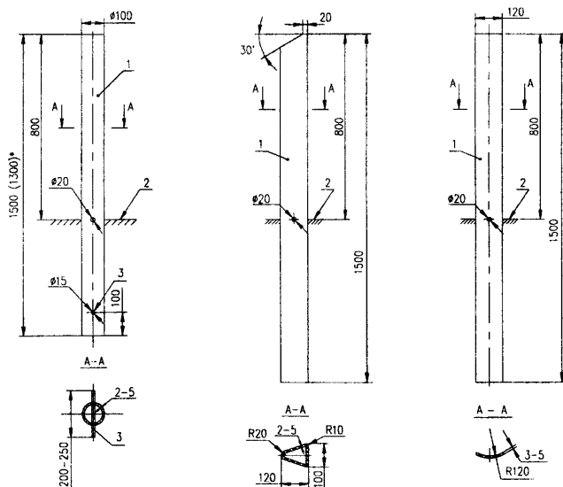
Рис. 1. Форма и размеры сплошных ударобезопасных сигнальных столбиков из композиционных материалов: 1 – корпус столбика; 2 – поверхность земли; 3 – анкерное устройство
