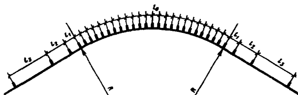
Рис. 9. Установка сигнальных столбиков в пределах кривых в продольном профиле
