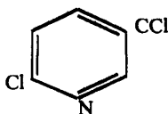
2-хлор-5-трихлорметилпиридин (2-хлор-5-ТХМП)
